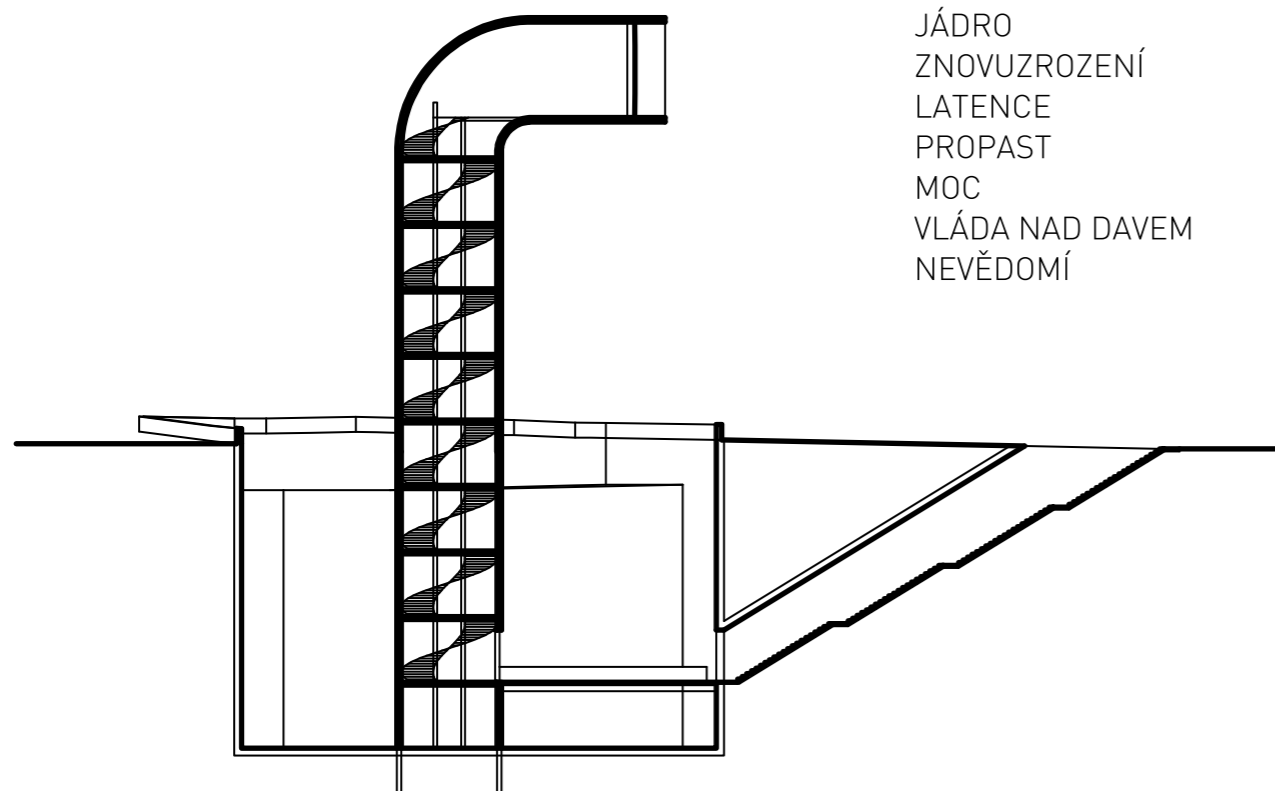
PŮDORYS, ŘEZ 1:500
