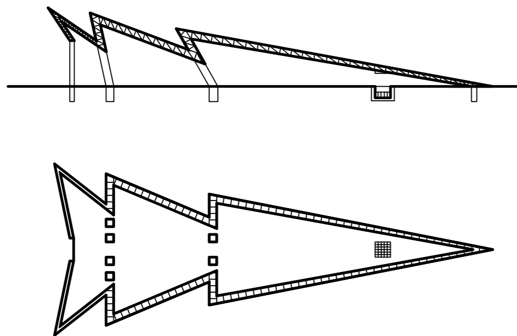
PŮDORYS, ŘEZ 1:500
