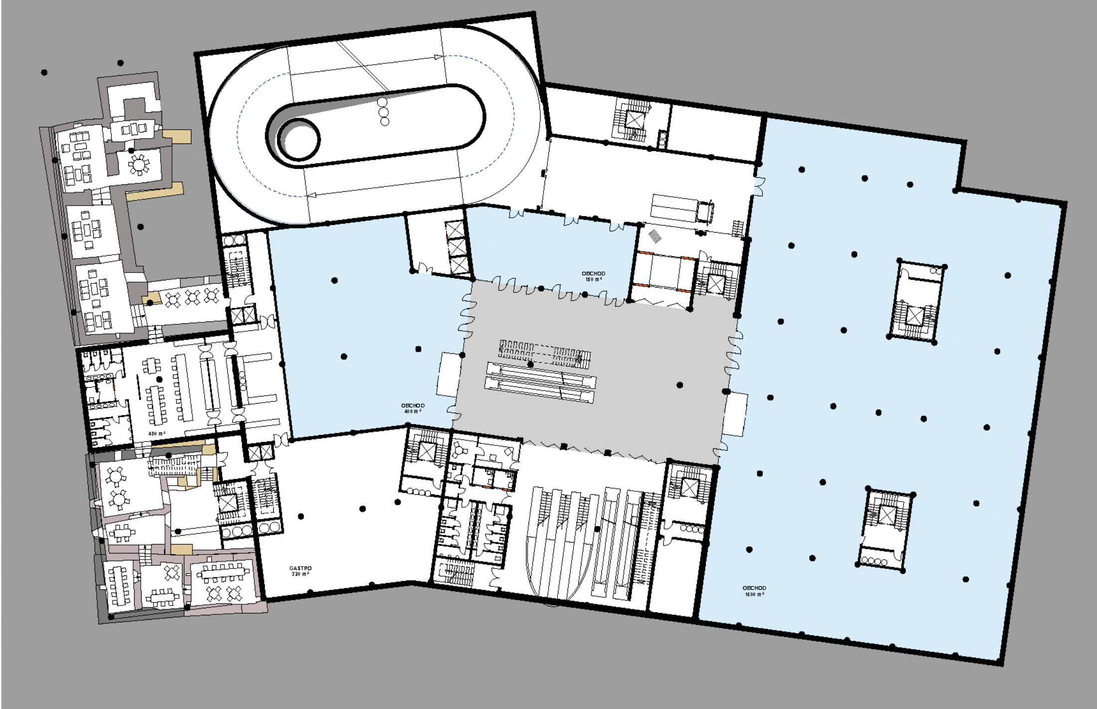
1. PP 1:400 VESTIBUL METRA A OBCHODNÍ PASÁŽ
