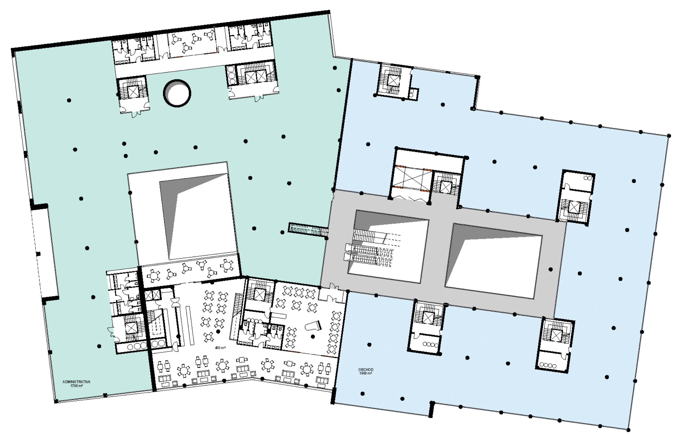
2. NP 1:400 ADMINISTRATIVA, OBCHOD A SLUŽBY
