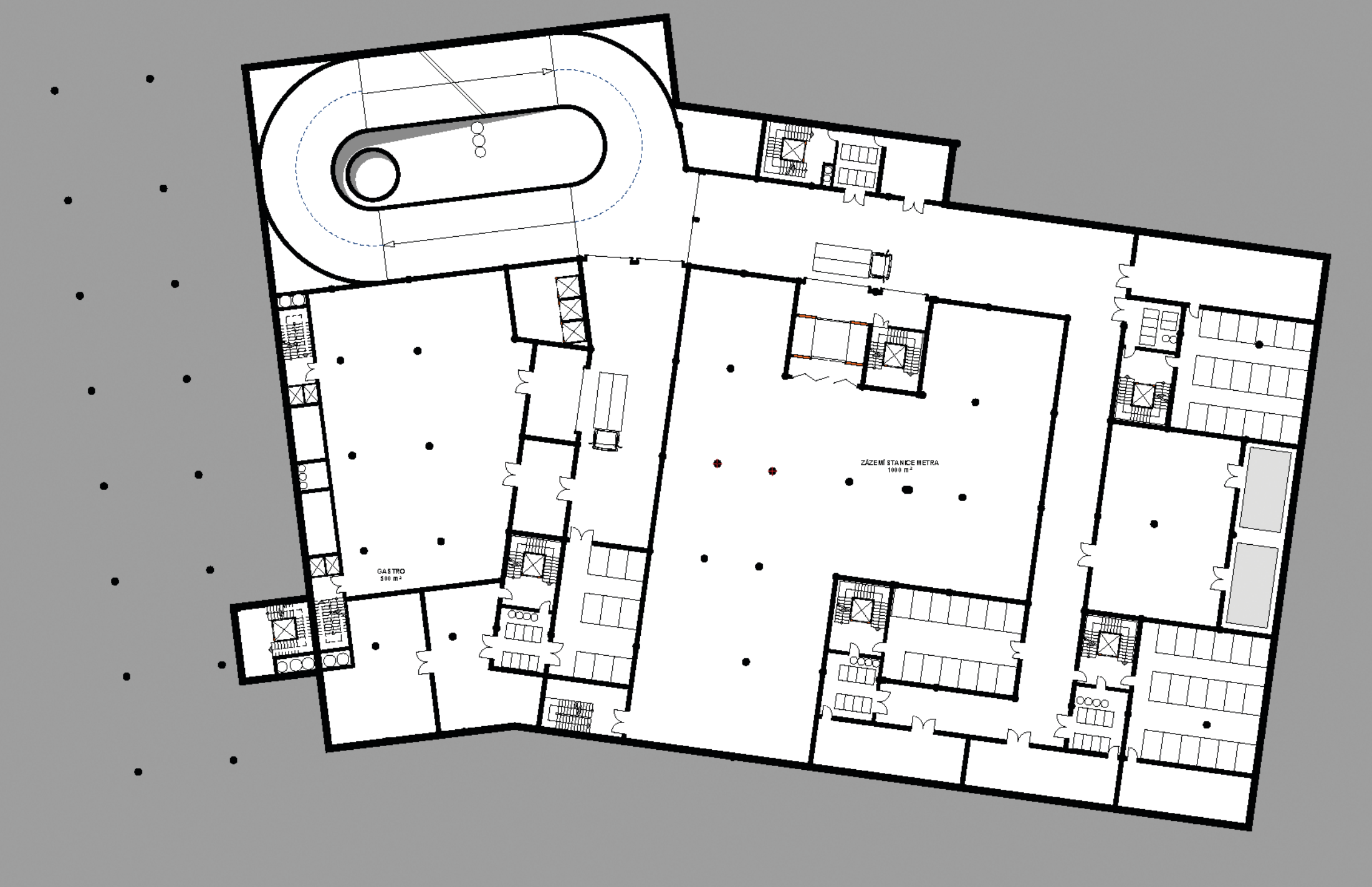
2. PP 1:400 SERVISNÍ PODLAŽÍ
