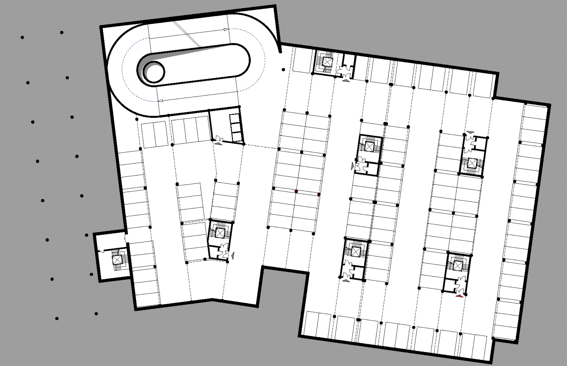
3. PP GARÁŽ RESIDENTŮ
