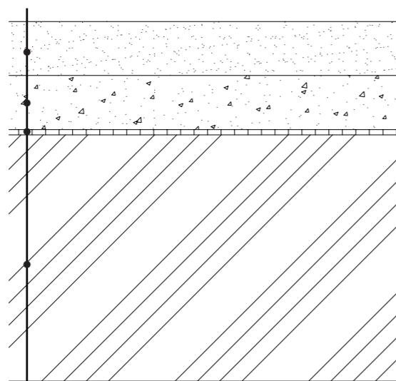
MLATOVÁ CESTA 1:15
