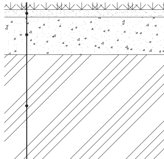
POBYTOVÝ TRÁVNÍK 1:15
