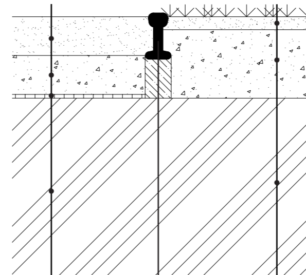
DETAIL PŘECHODU MEZI MLATOVOU CESTOU A TRÁVNÍKEM 1:15
