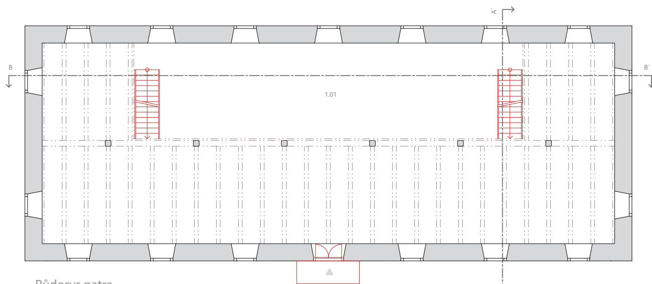
Půdorys patra
