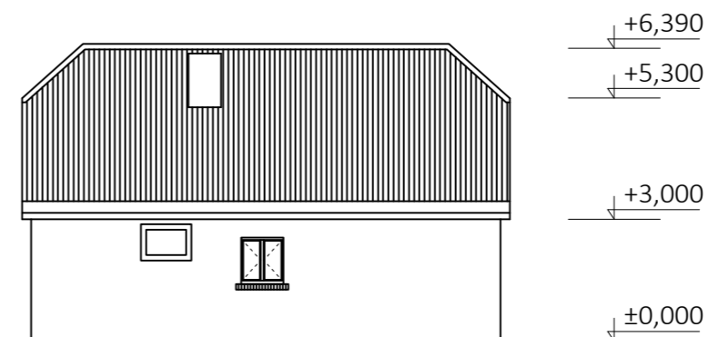
VÝCHODNÍ FASÁDA
