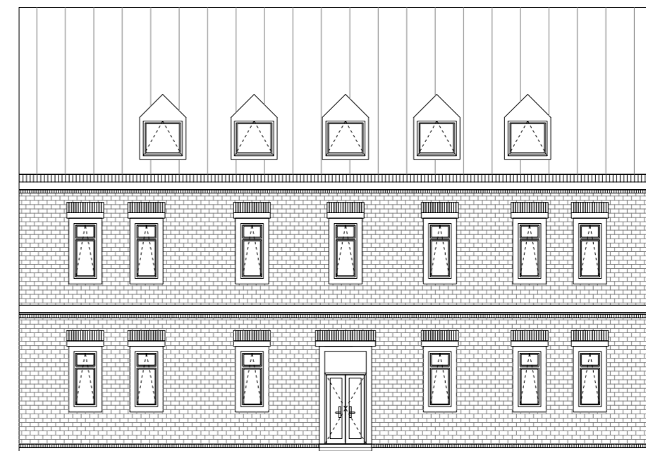
JIHOVÝCHODNÍ FASÁDA
