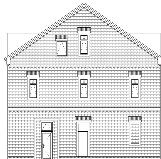
SEVEROVÝCHODNÍ FASÁDA
