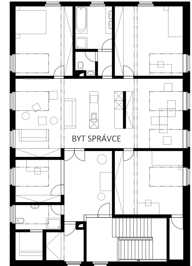
PŮDORYS DRUHÉ PATRO
