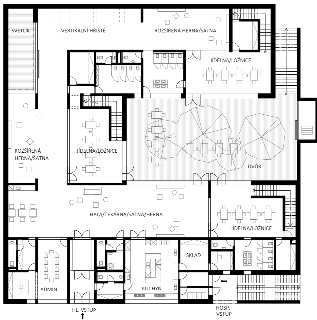
PŮDORYS PP
