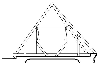
ŘEZ B-B' SEVERNÍ KŘÍDLO_RENESANČNÍ KROV_PLNÁ VAZBA
