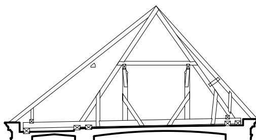
ŘEZ F-F' JIŽNÍ KŘÍDLO_BAROKNÍ KROV_PLNÁ VAZBA
