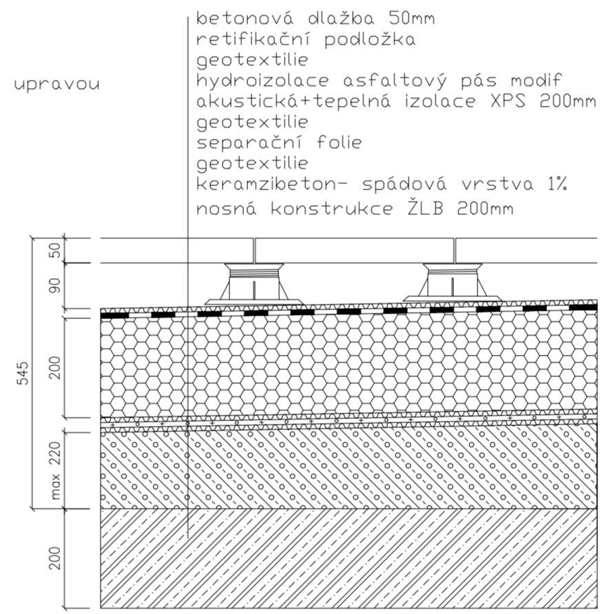
S3 pochozí střecha
