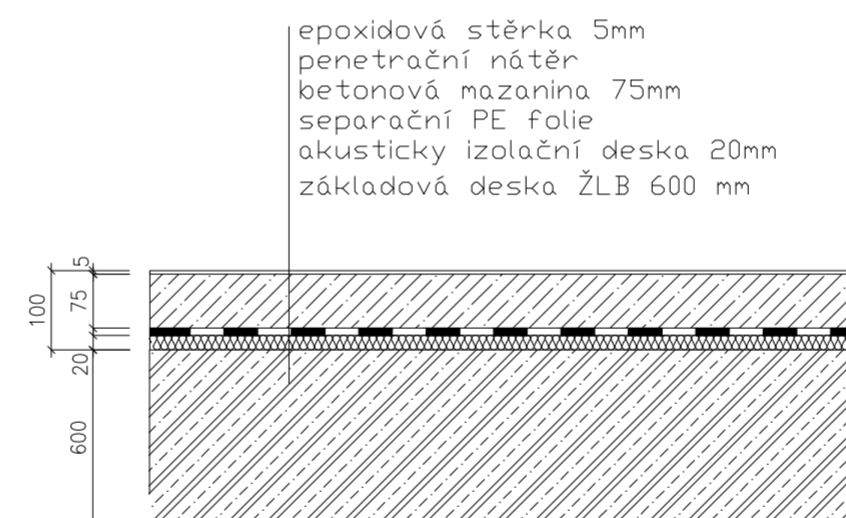
P6 technická místnost/ garáž
