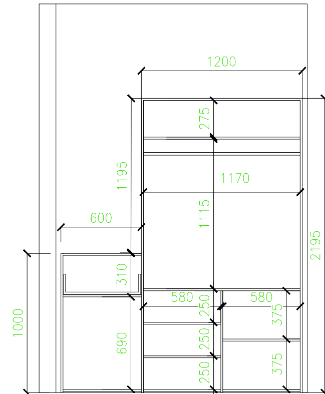
ŘEZ SKŘÍŇE PODÉLNÝ
