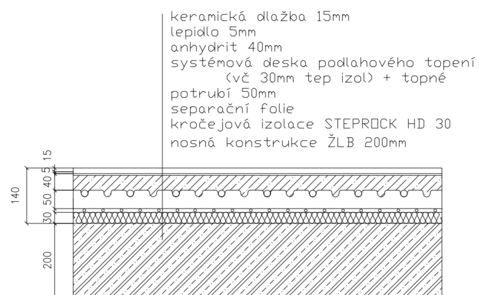
P2 byt- koupelna/WC
