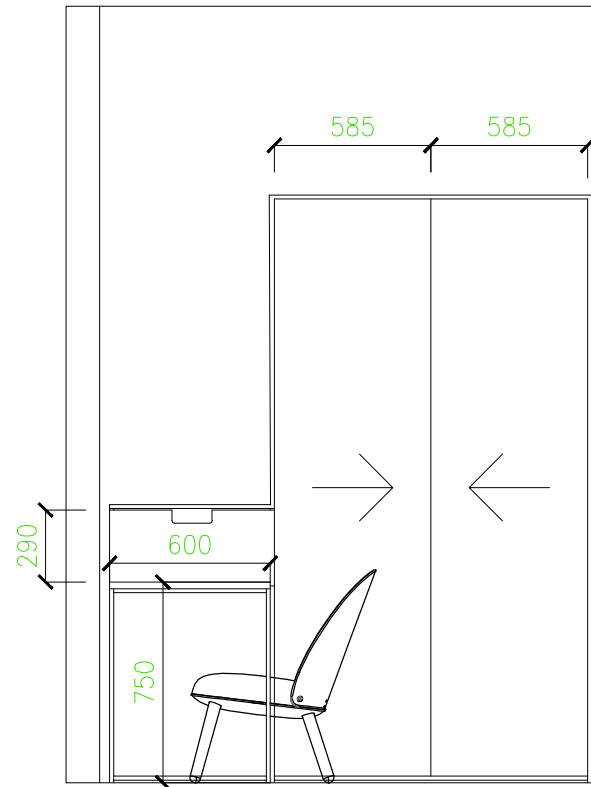
POHLED JIŽNÍ, NA SKŘÍŇ
