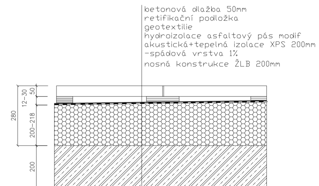
P7 zateplená lodžie
