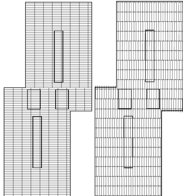
Schéma umístění nosníků, stojek (1) a bednicích desek (2)
