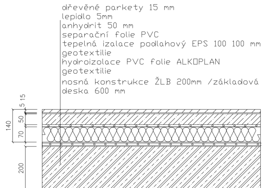
P5 knihovna 2NP
