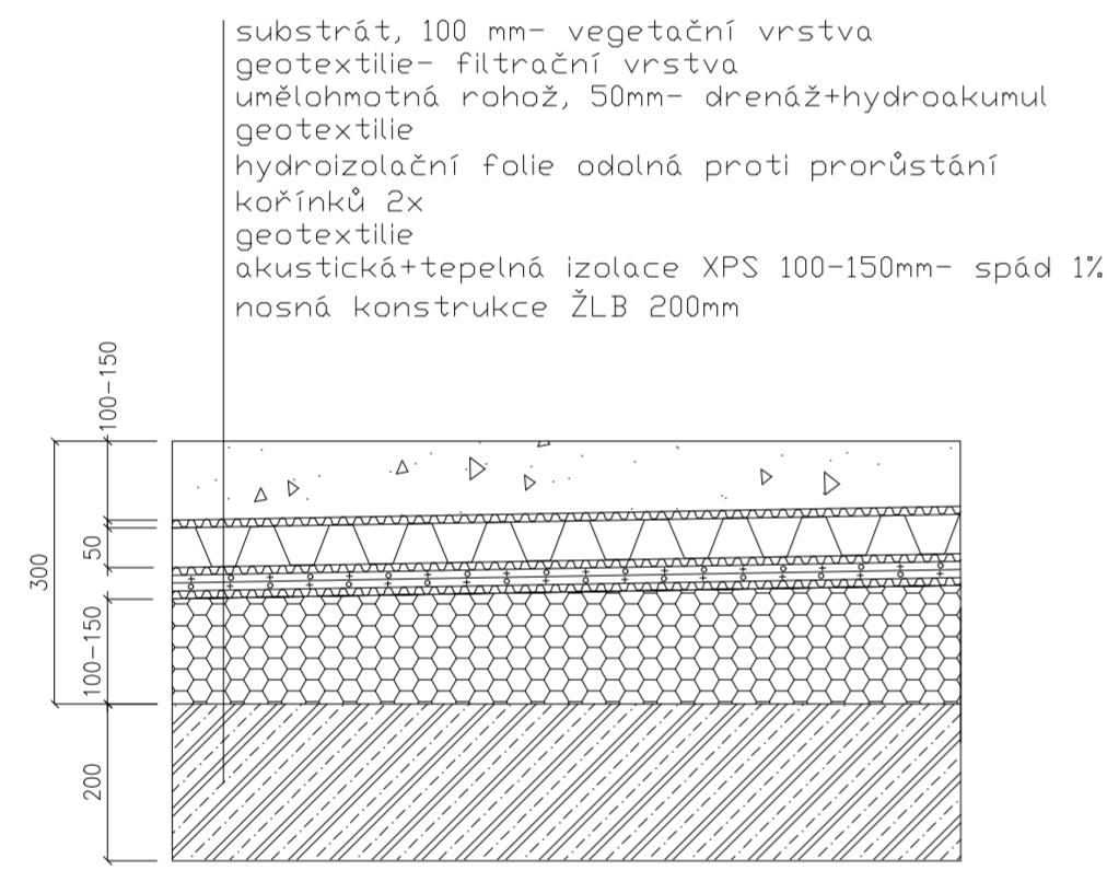
S1 pochozí střecha nad podzemní garáží
