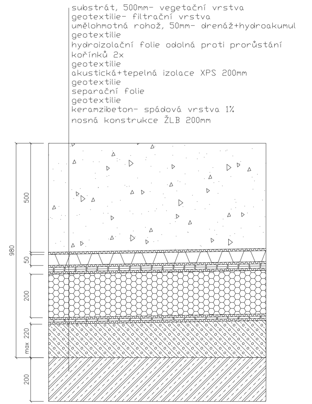
S4 střecha s extenzivní zelení
