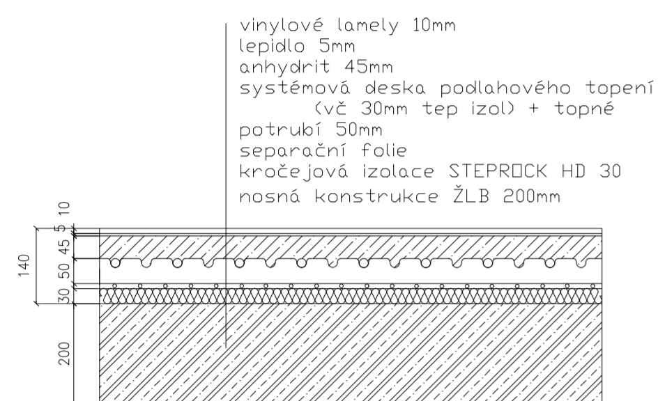
P1 interier bytu
