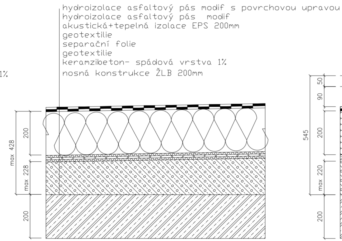
S2 nepochozí střecha
