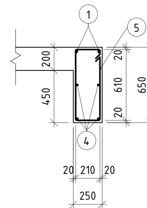
ŘEZ A-A
