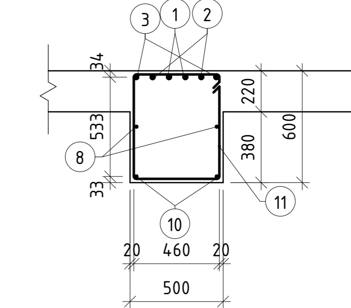
ŘEZ C-C
