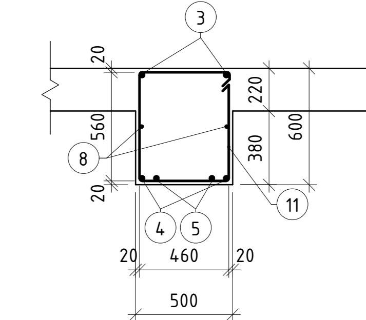
ŘEZ B-B
