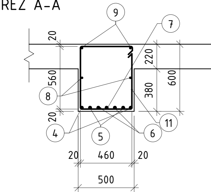
ŘEZ A-A
