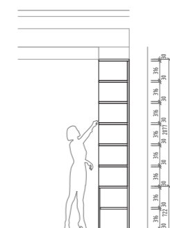
ŘEZ 1-1
