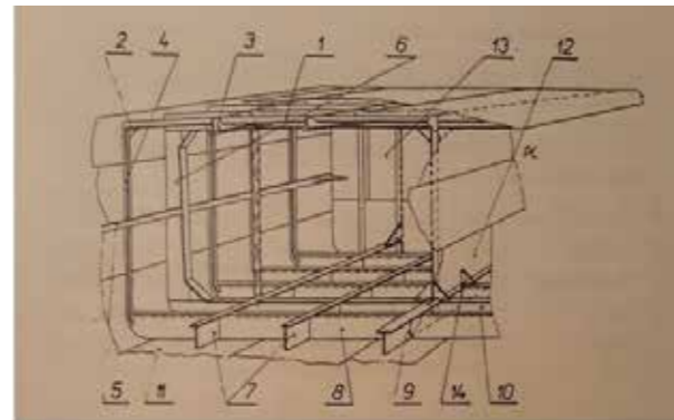
obr.5: Části příčného vyztužení trupu. 1.- palubník, 2.- rožnice 3.- podvlak, 4.- žebro, 5.-bočnik (stringer), 6.- rámové žebro, 7.- postranní páteř, 8.- plná příčka, 9.- střední páteř, 10.- rámová příčka, 11.- dnová obšívka, 12.- příčná přepážka, 14.- rožnice přepážky
