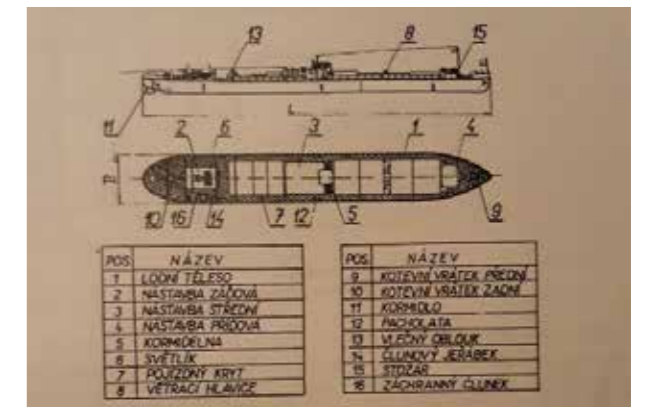
obr.3: Hlavní části lodního tělesa
