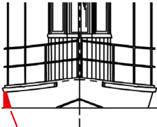
Chybějící výtlač, malá stabilita
