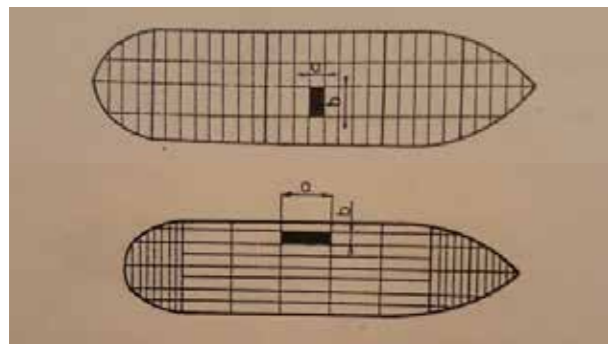
obr.4: příčná soustava (nahore), podélná soustava (dole)
