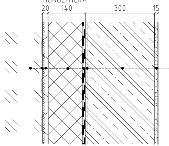
S02 STĚNA OBVODOVÁ SUTERÉN, MONOLITICKÁ
