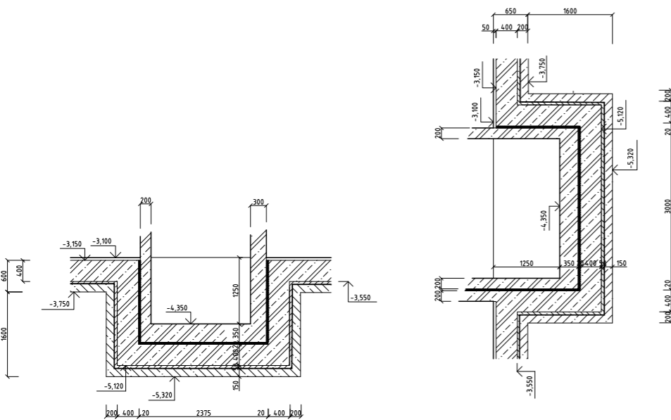
Detail DET1 Výtahová šachta M 1:50
