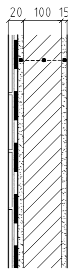
S11 PŘÍČKA KOUPELNA
