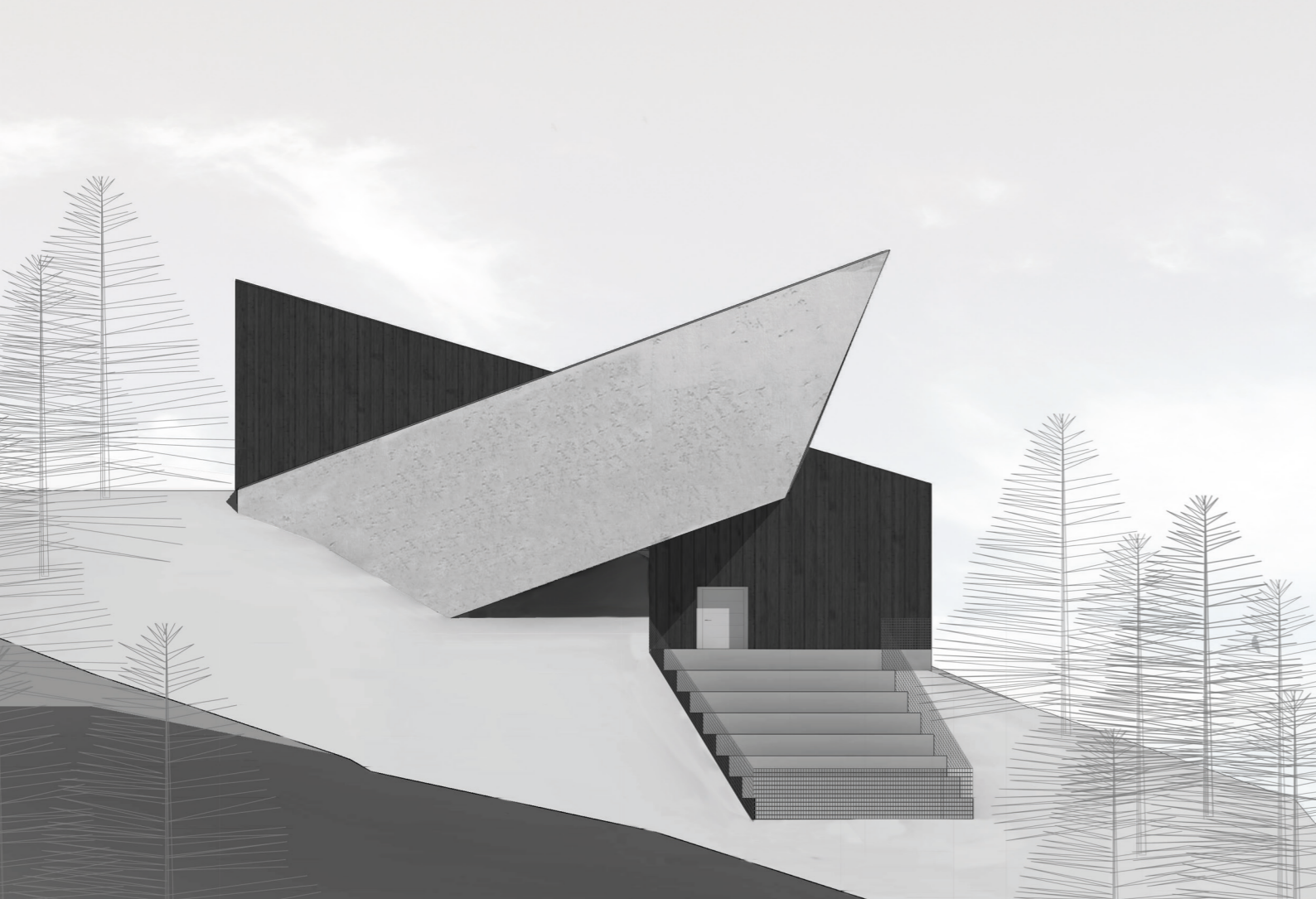
POHLED JIŽNÍ 1:200 POHLED VÝCHODNÍ 1:200 ŘEZ A - A 1:150
