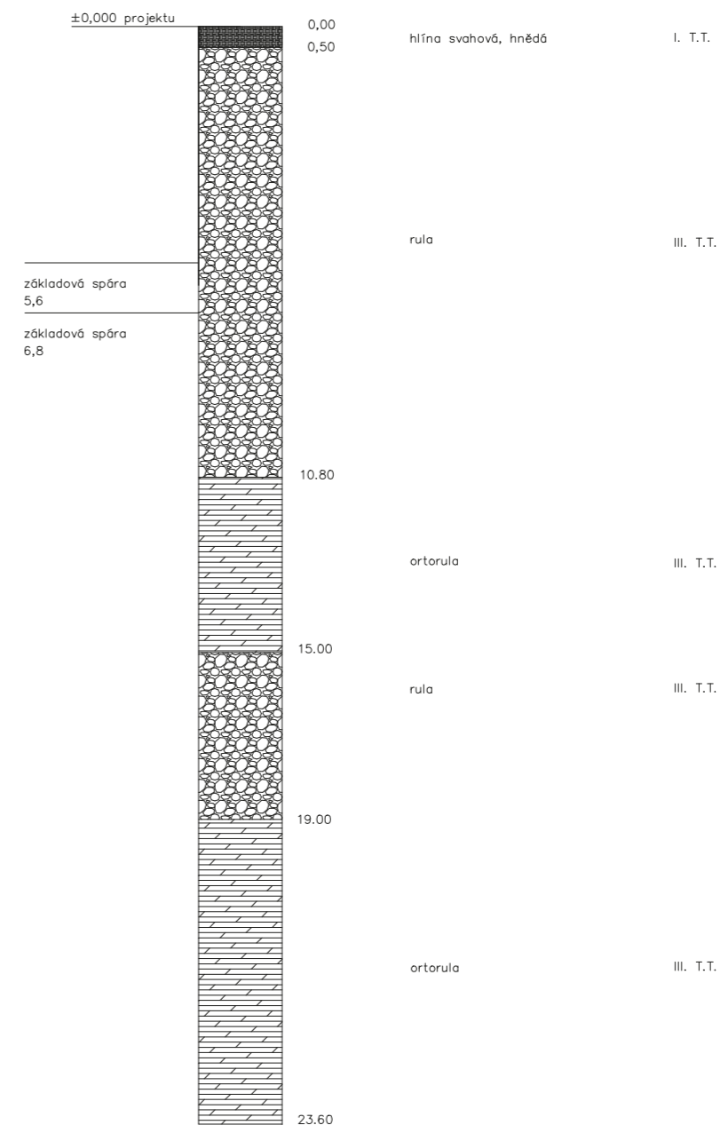
GEOLOGICKÝ PROFIL
