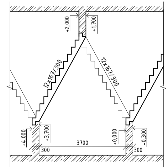
ŘEZ SCHODIŠTĚVÝM RAMENEM SR1
