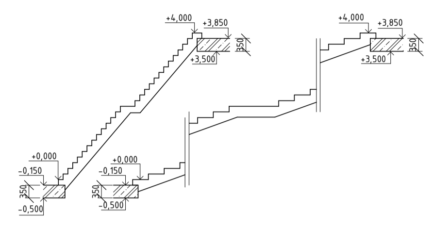
ROZVINUTÝ ŘEZ SCHODIŠTĚVÝM RAMENEM SR2
