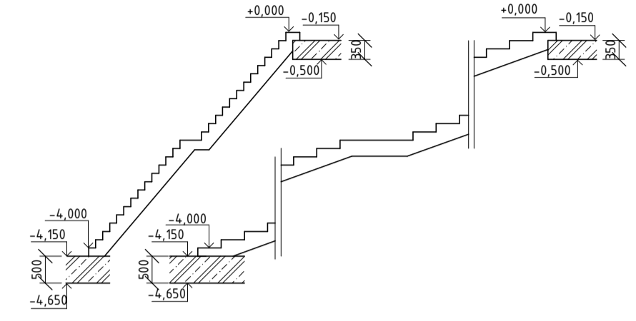
ROZVINUTÝ ŘEZ SCHODIŠTĚVÝM RAMENEM SR2
