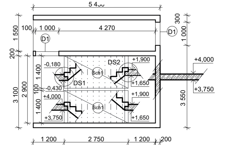
DS1 1:50
