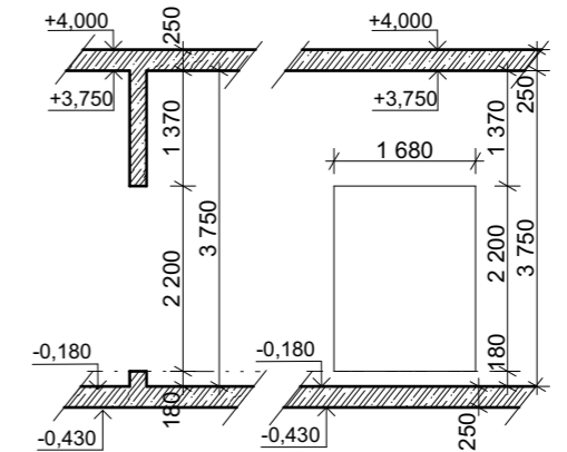
D3 1:100
