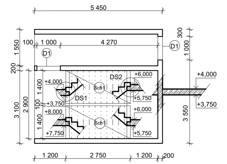
DS4 1:100
