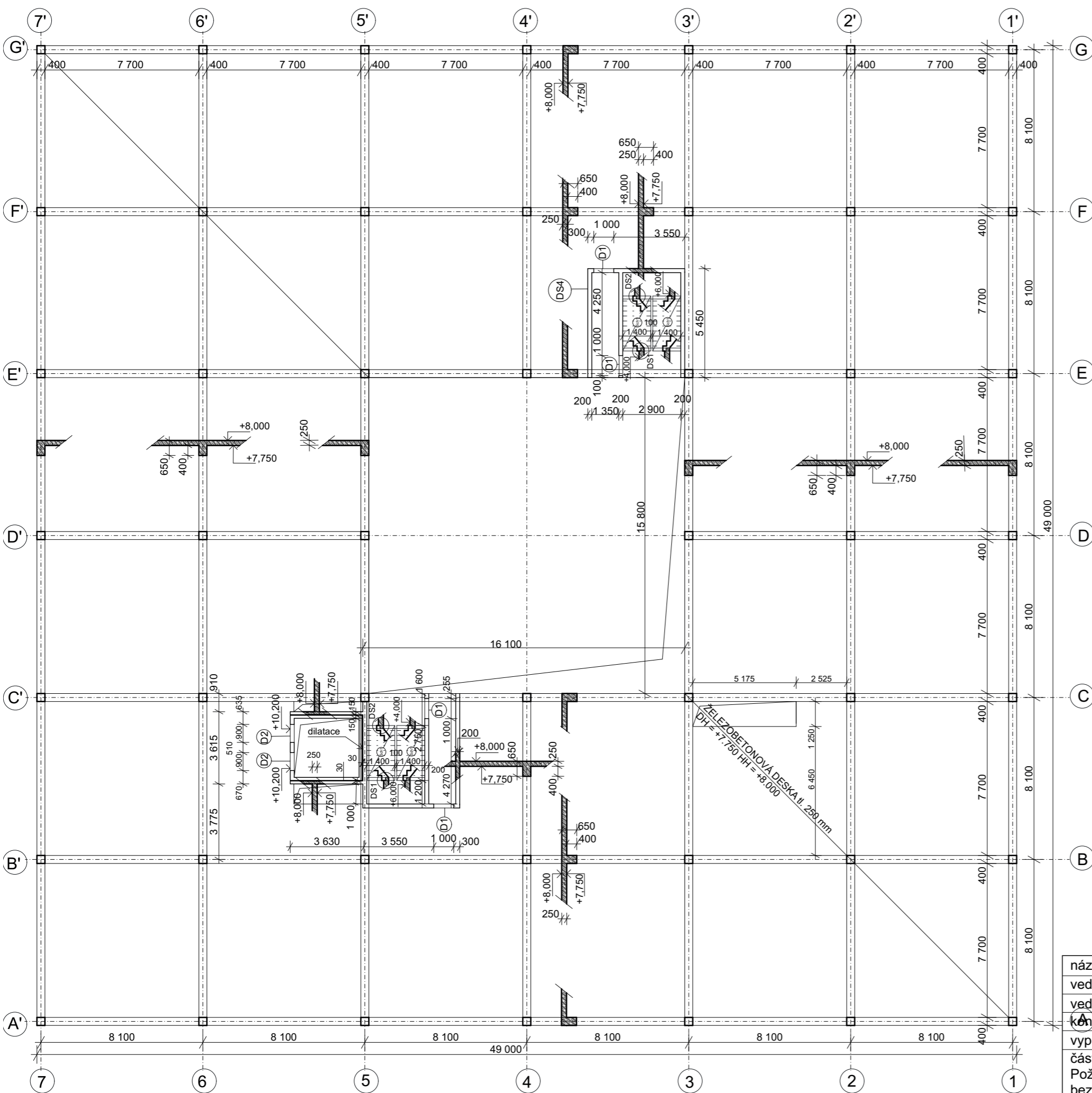
D2 1:100
