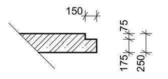
DS2 1:50
