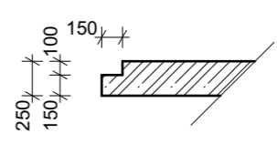
DS1 1:50
