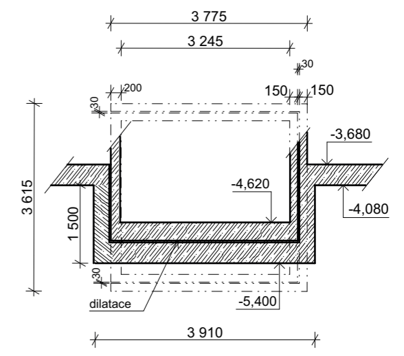
D3 Výtahová šachta 1:100
