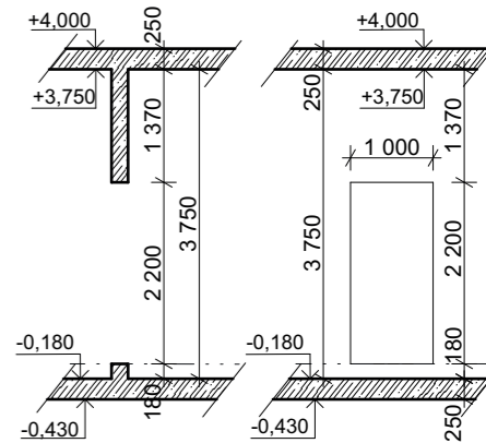
D1 1:100
