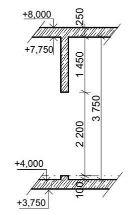
D2 1:100
