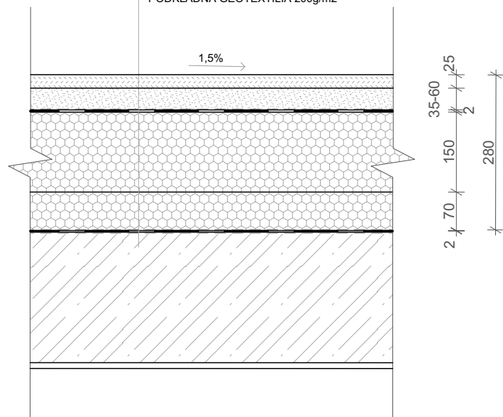
PAVLAČ NAD KULTÚRNYM CENTROM
