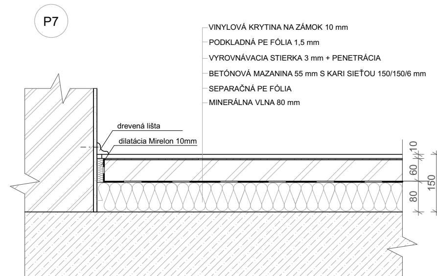
PREDSIENĽ
