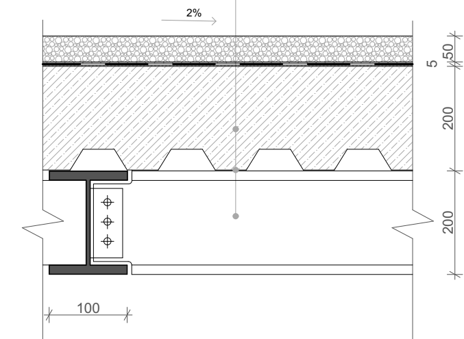
PAVLAČ STRECHA
