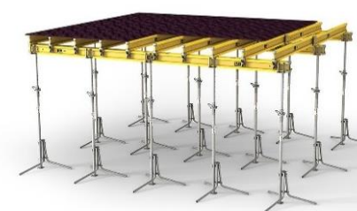
debnenie stropu
