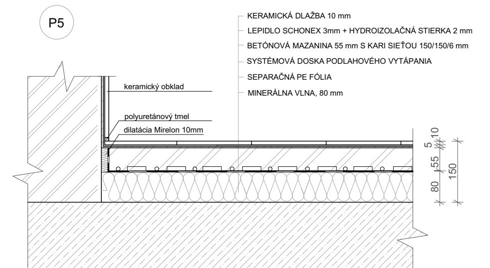
HYGIENICKÉ ZÁZEMIE
