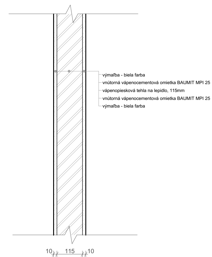
S8 SKLADBA PRIEČKY KULTÚRNE CENTRUM, BYTY
