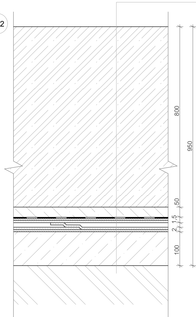
SKLADBA ZÁKLADOVEJ VANE
