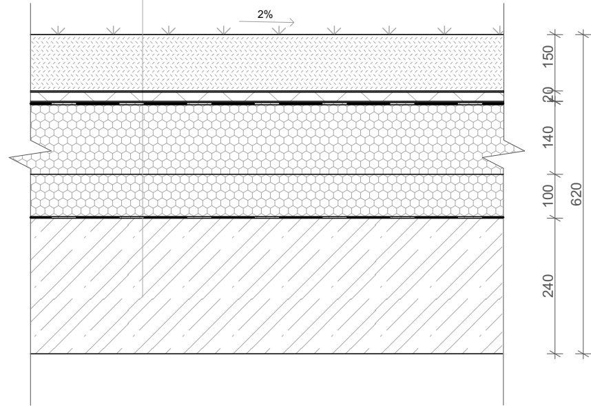
ZASTREŠENIE GARÁŽI
