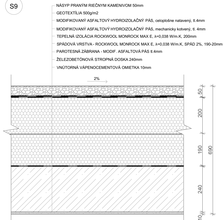
PLOCHÁ NEPOCHÔDZNA STRECHA
