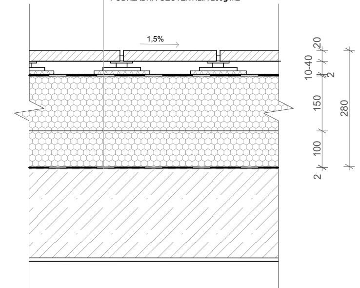
PAVLAČ NAD KULTÚRNYM CENTROM
