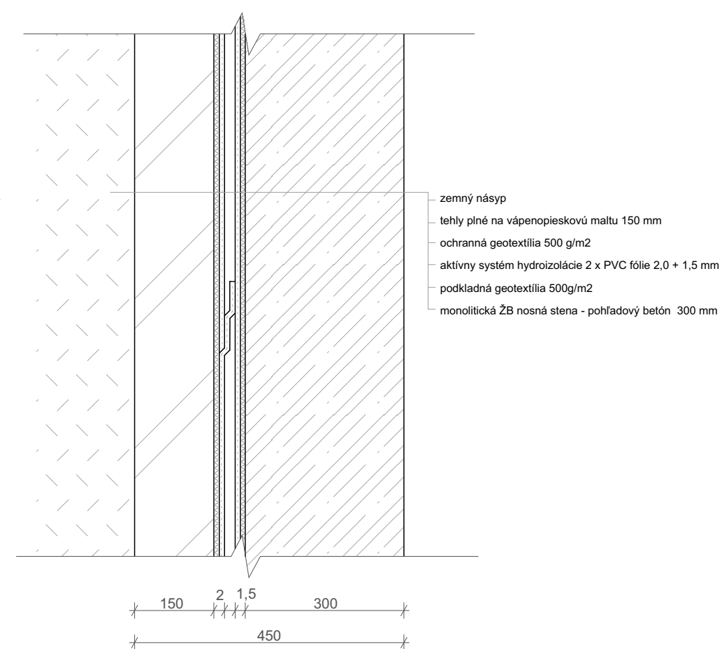
S3 SKLADBA STENY SUTERÉN POD ZÁMRZNOU HĽBKOU
