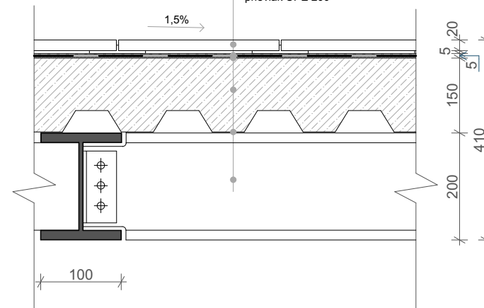
PAVLAČ PODLAHA
