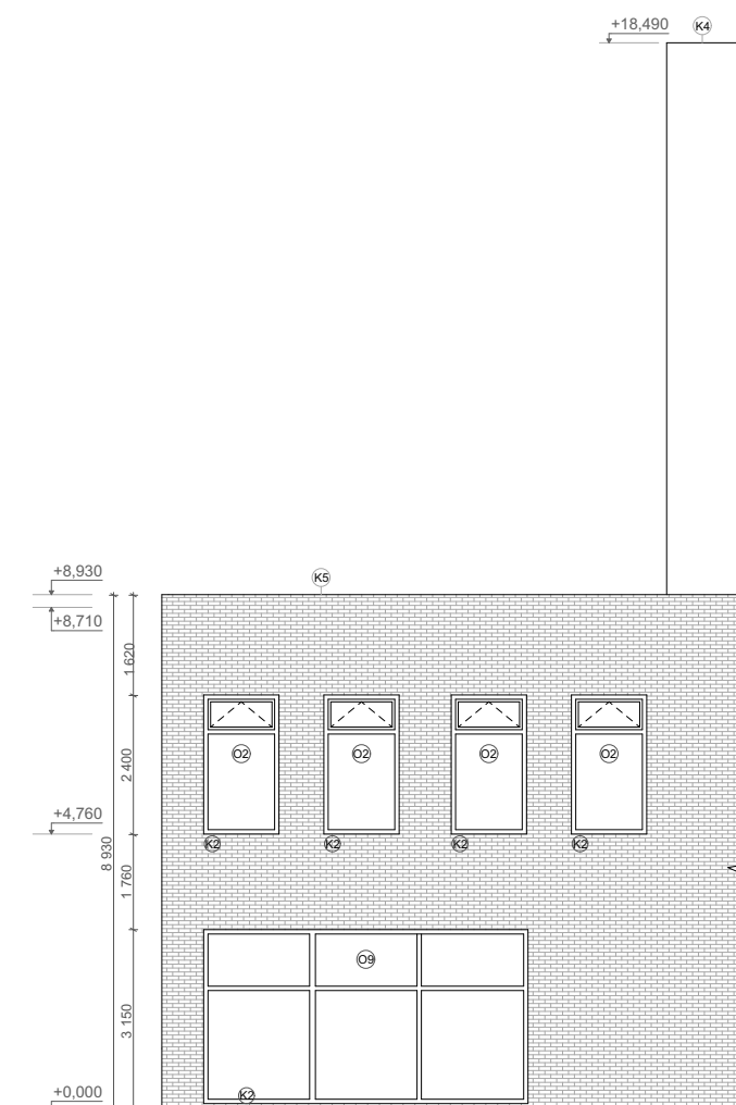
POHĽAD VÝCHODNÝ - VNÚTROBLOK
