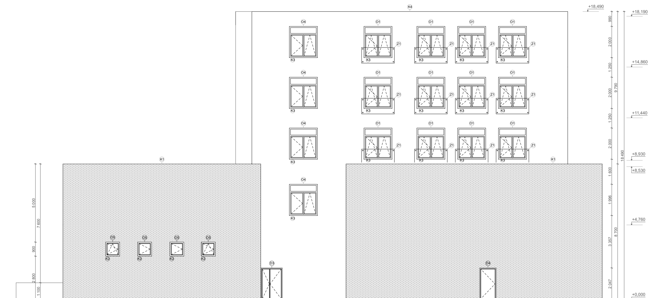
POHĽAD VÝCHODNÝ
