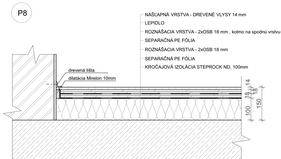
SPOLOČENSKÁ SÁLA
