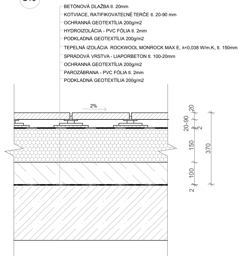
TERASA NAD GARÁŽAMI
