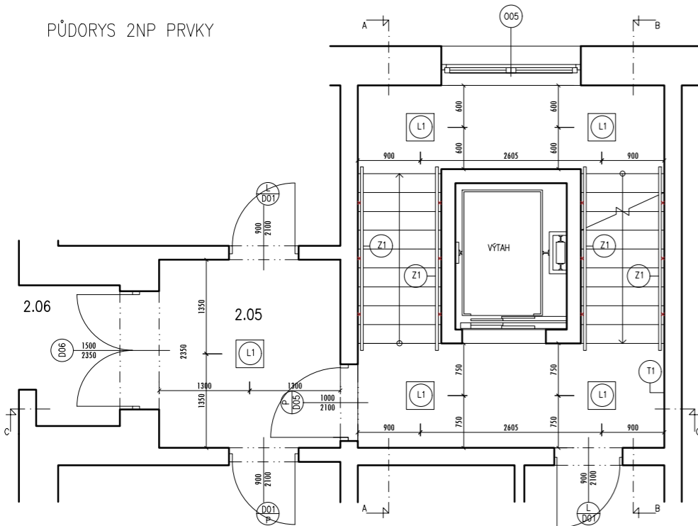
PŮDORYS 2NP POVRCHY
