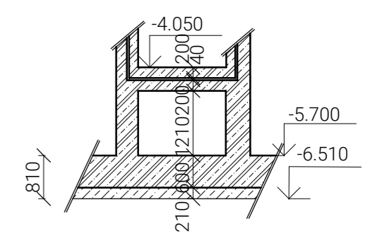
Řez A-A
