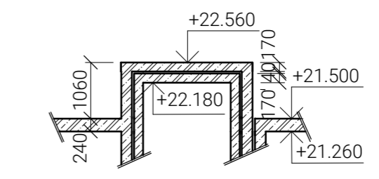
ŘEZ B-B
