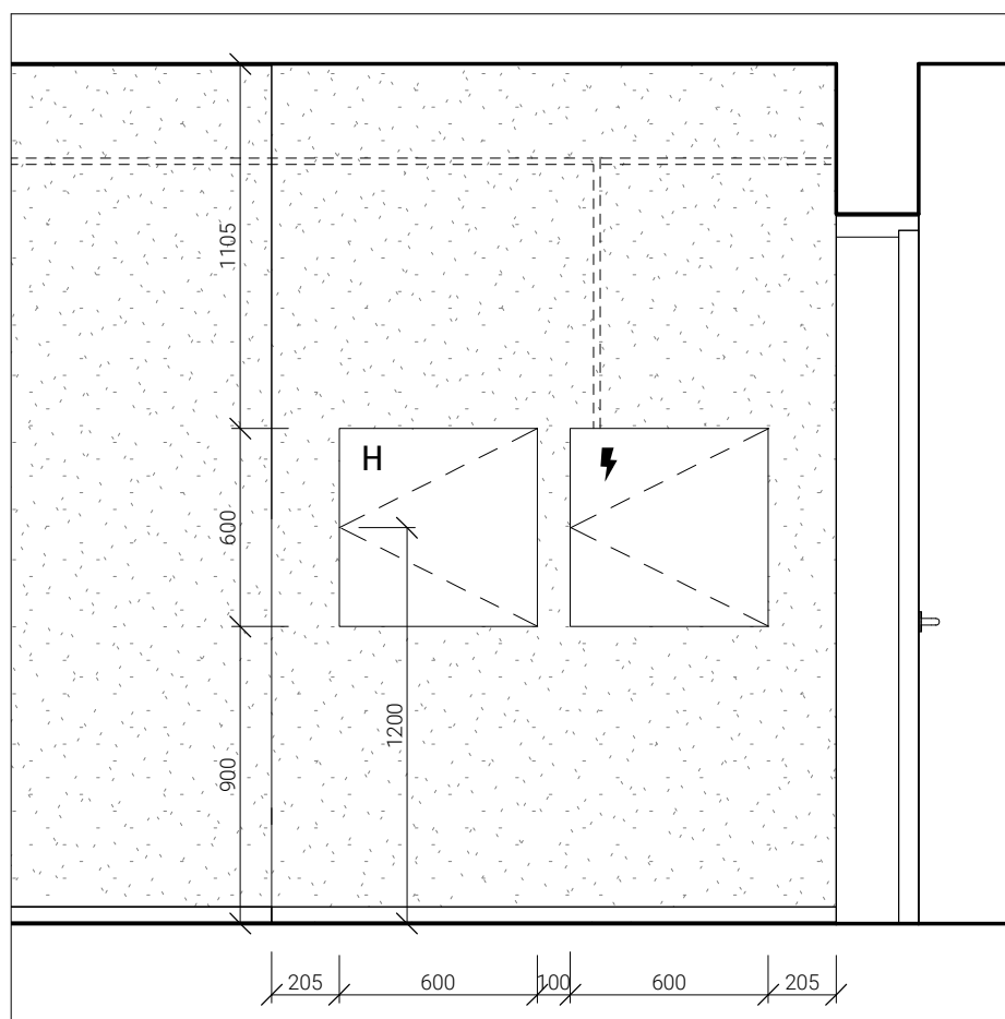
Pohled B
