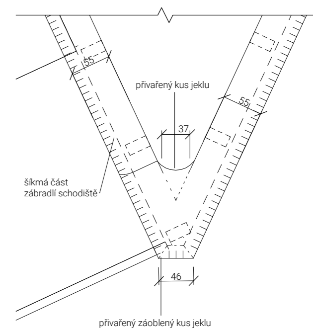
Detail F madlo zábradlí
