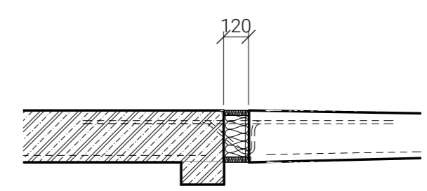
DETAIL ISO NOSNÍKU ISOKORB XT K v.240 tl.120 mm
