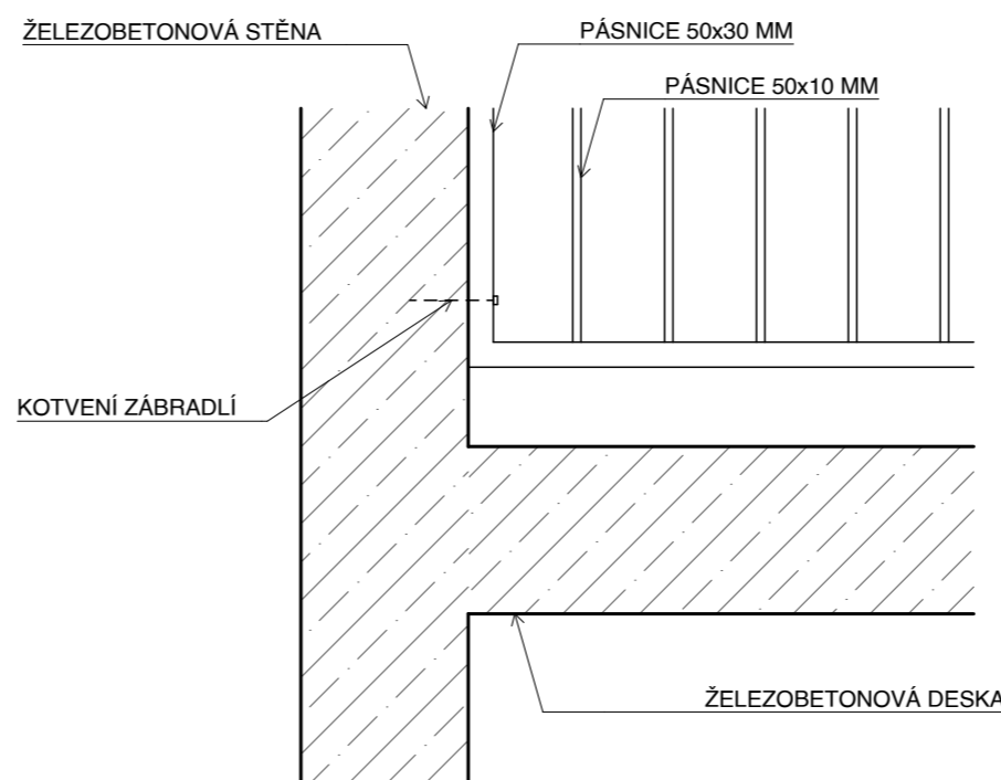
kotvení zábradlí do stěny/sloupu
