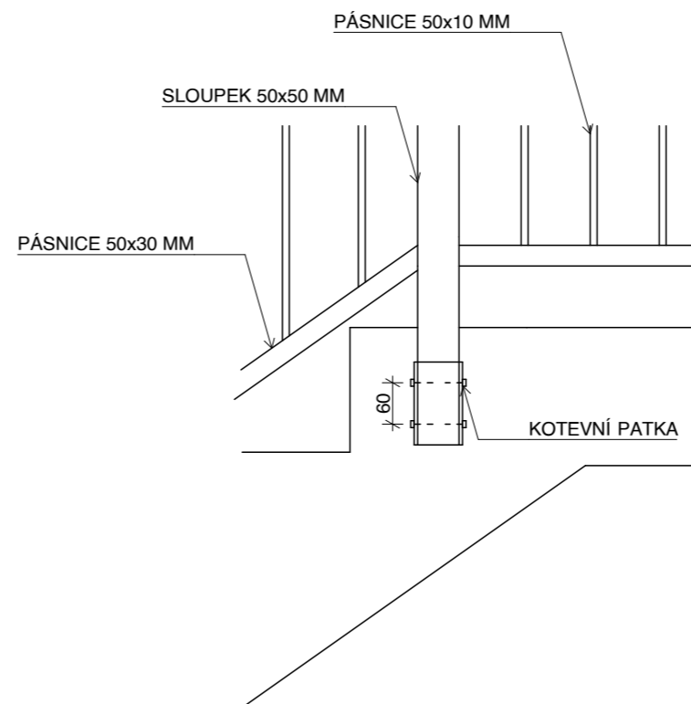
kotvení sloupku do schodiště - pohled z boku
