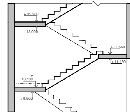
POHLED P1:
