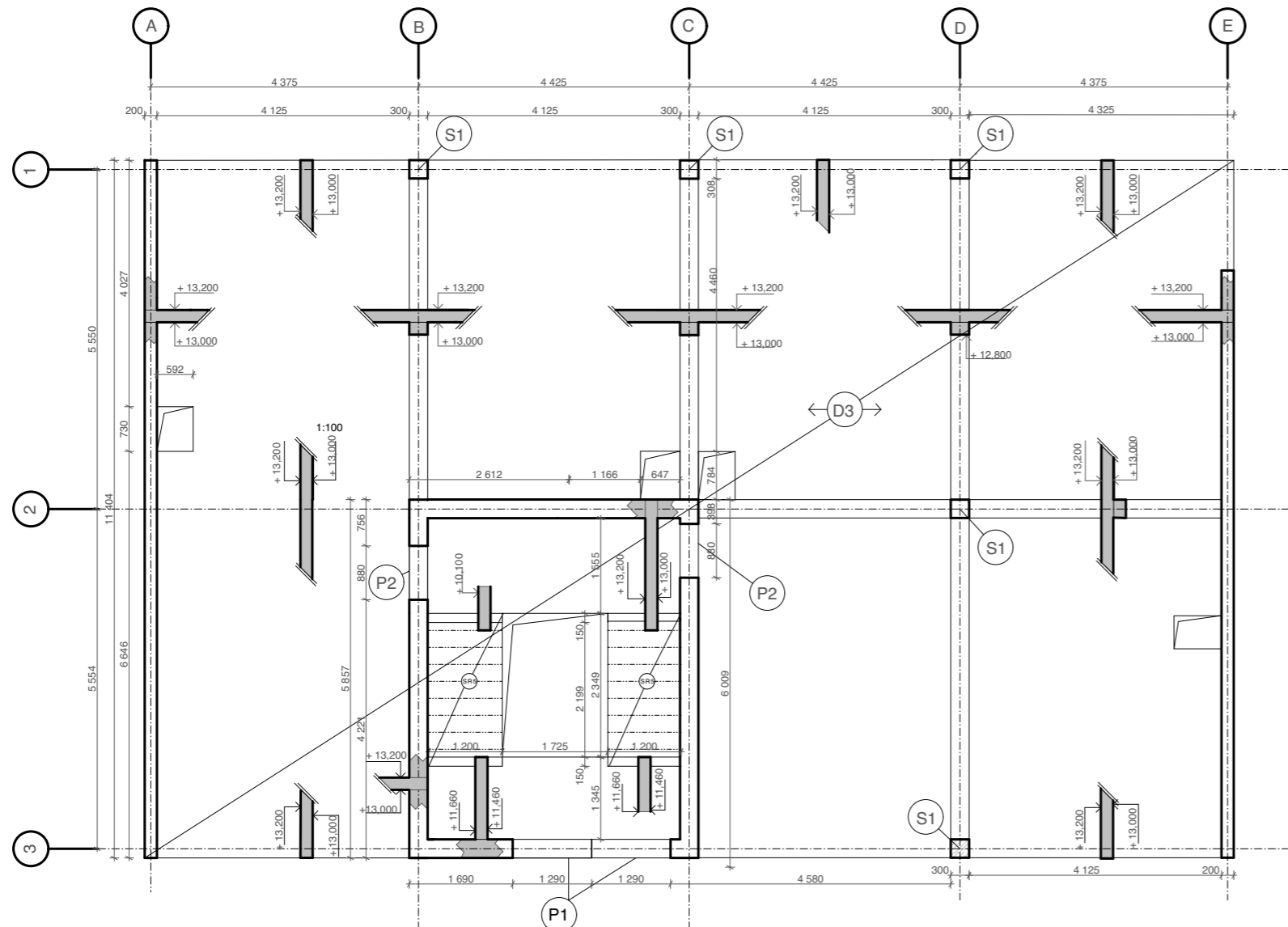
POHLED P1:
