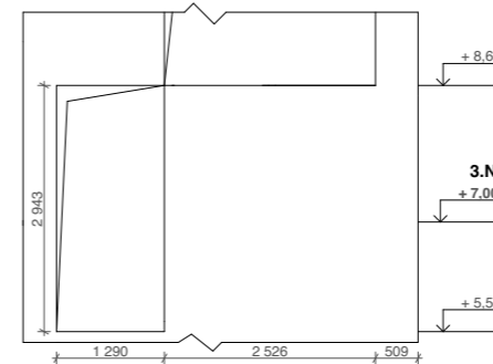
POHLED P1:
