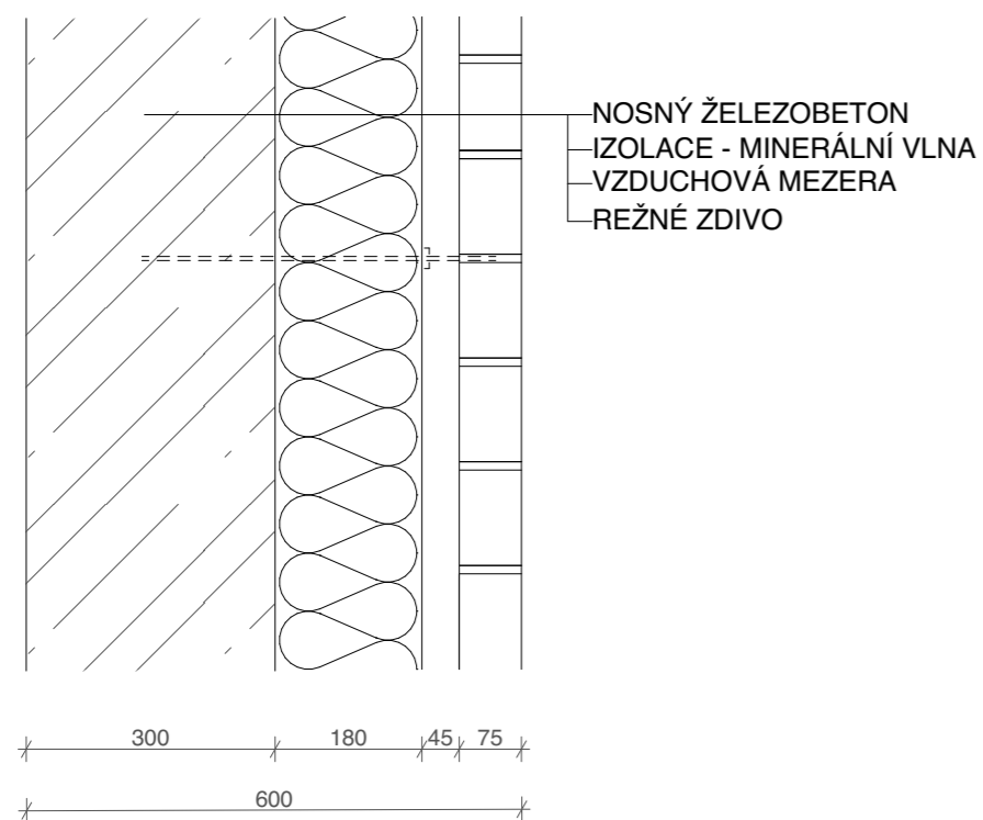
S04 SKLADBA NOSNÉ STĚNY TUBUSU KOLEM SCHODIŠTĚ - NÁVAZNOST S EXTERIÉREM
