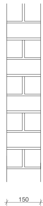
S06 ZDĚNÉ PŘÍČKY
