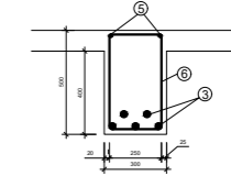
ŘEZ C-C'
