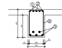
ŘEZ C-C'
