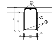
ŘEZ B-B'
