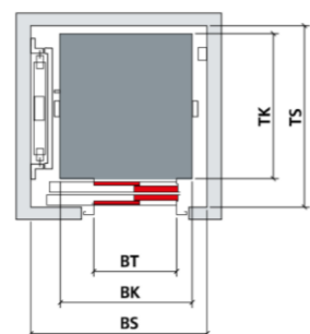
Kabina s jedním vstupem
