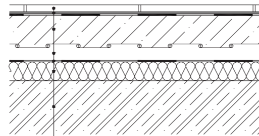
P2 Byty - koupelny, WC
