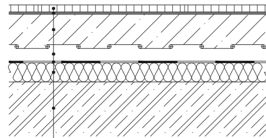
P1 Byty - ložnice, obývací pokoje
