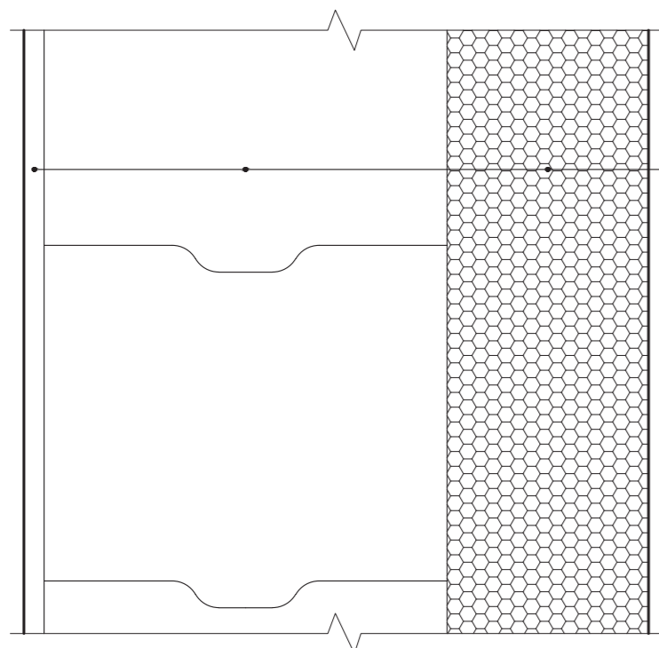
S4 Sdružená stěna se sousedem
