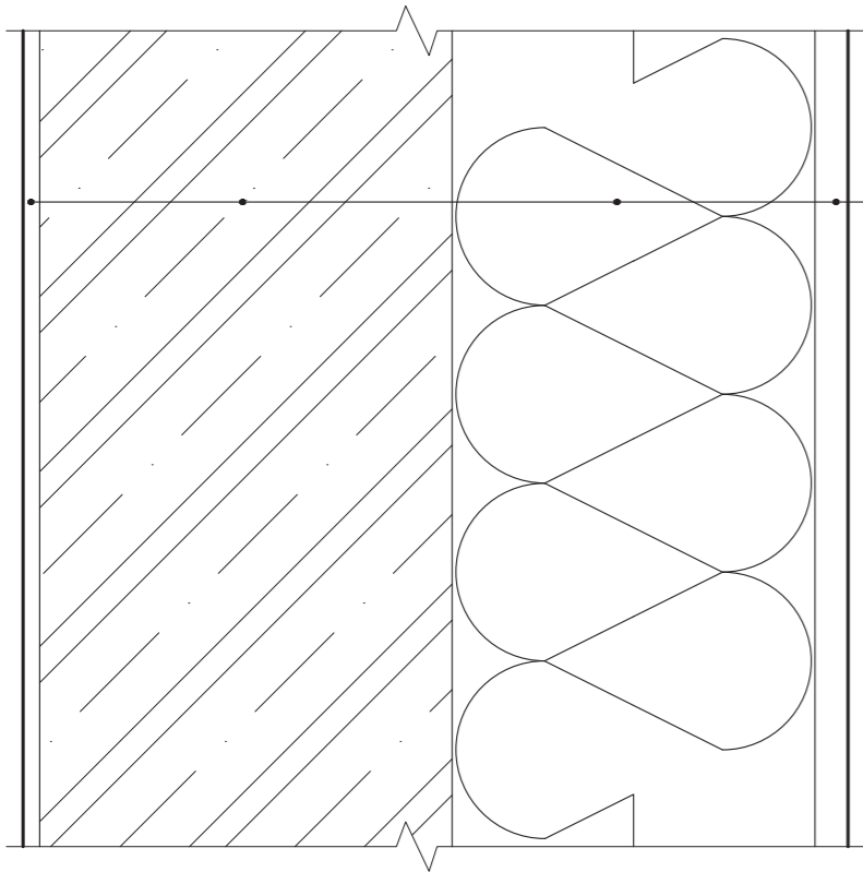
S1 Obvodové stěny
