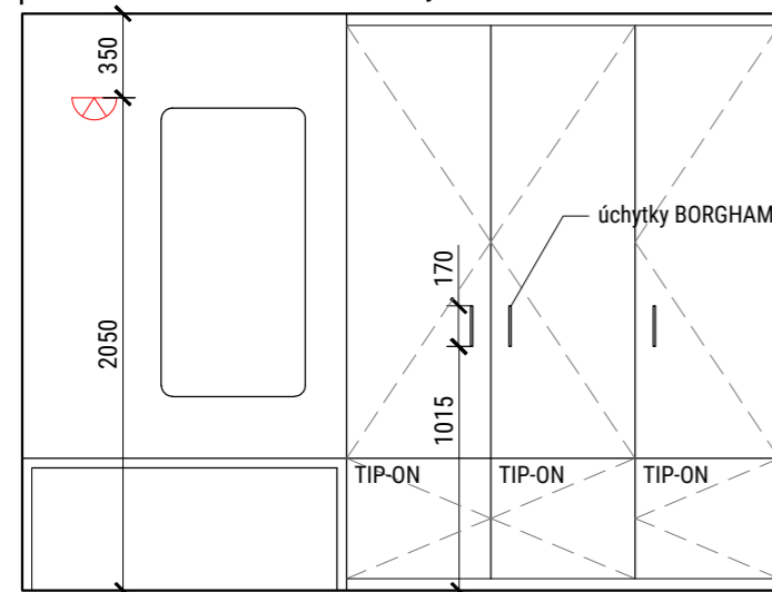
pohled A nábytek A - šatní skříň
