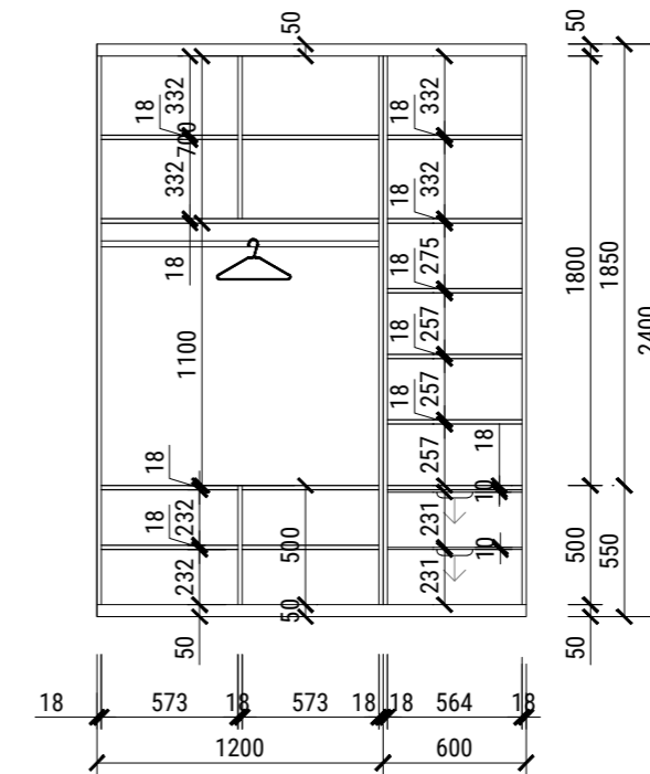
nábytek A - šatní skříň
