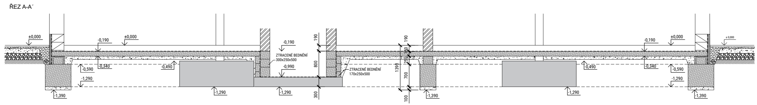
ZÁKLADY ZDÍ NA NÁDVORÍ VIZ. VÝKRES Č. D.1.B.13 : Výkres základů - objekt č.2
