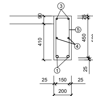
ŘEZ A-A" 1:25
