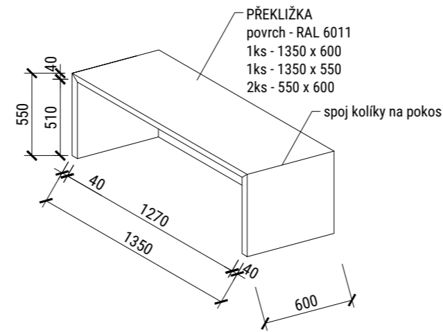
nábytek B - lavice
