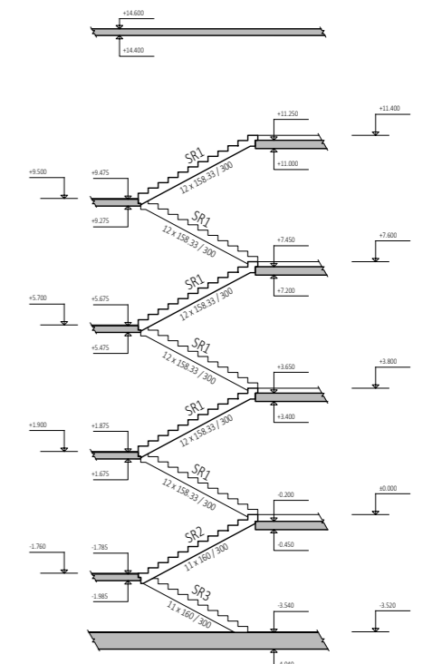
ŘEZ DVOURAMENNÝM SCHODIŠTĚM S PREFABRIKOVANÝMI RAMENY
