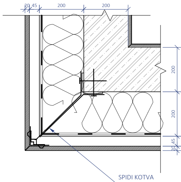
B PŮDORYS PROVEDENÍ KAMENICKÉHO ROHU
