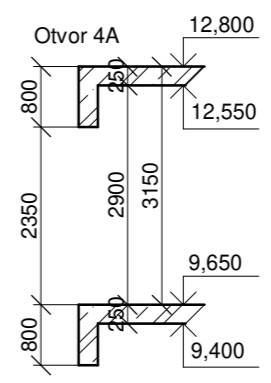
Řezy
