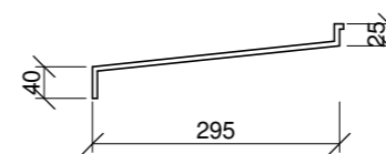
KP04 Okapní parapet Materiál: Titanzinek, tl. 0,6mm
