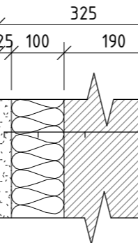
S9 - Obvodová stěna temperované úklidové místnosti
