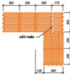
VAZBA ROHŮ A KOUTŮ
