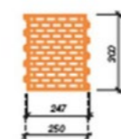
UKONČENÍ STĚNY NÍZKÝMI CIHLAMI (2/3 výškový modul - 167 mm)
