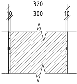
S10 - Interierová nosná stěna
