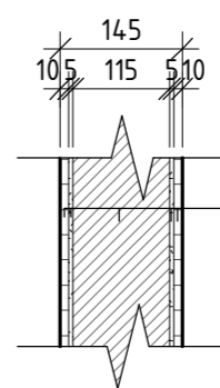
S11 - Vnitřní příčka mezi koupelnami
