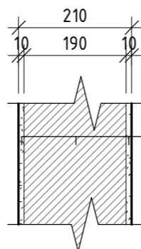
S6 - Akustická příčka mezi pokoji
