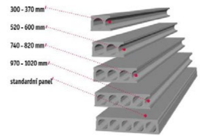
PANELY SPIROLL VÝŠKY 265 mm
