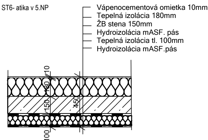
ST6- atika v 5.NP
