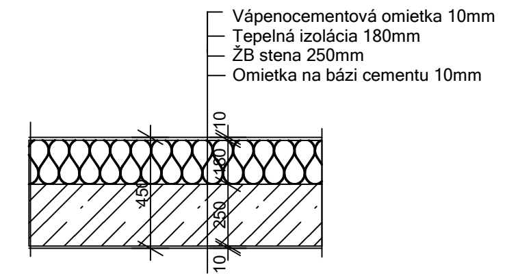
ST4- nosná obvodová stena v 1.NP
