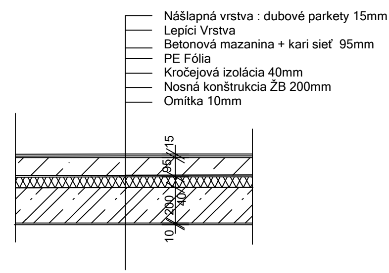
P3- podlaha vo vstupných priestoroch bytov
