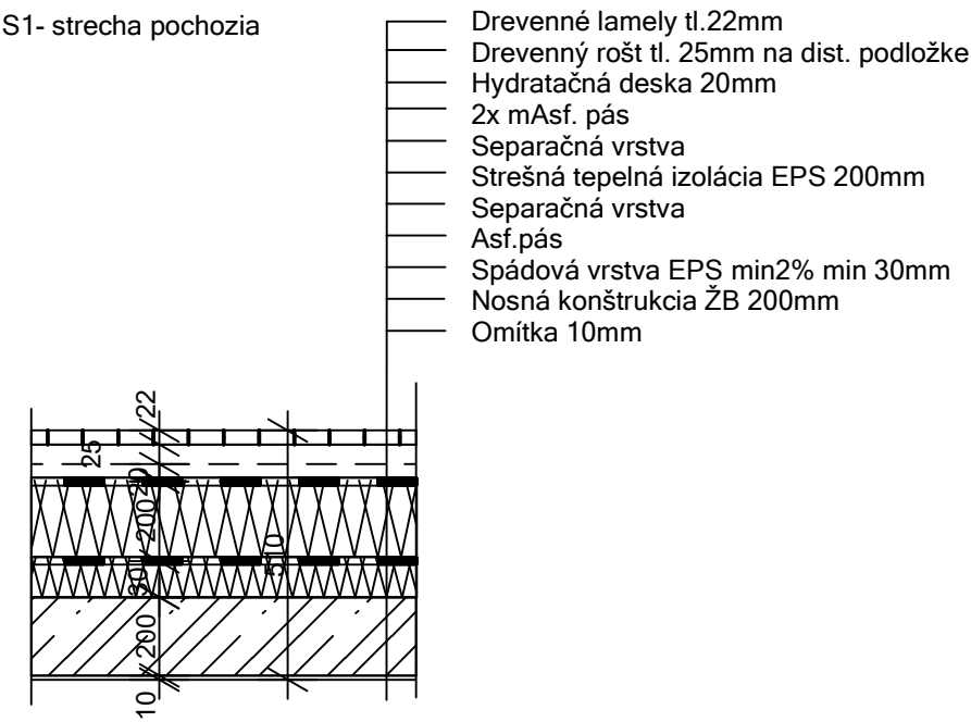
S1- strecha pochozia
