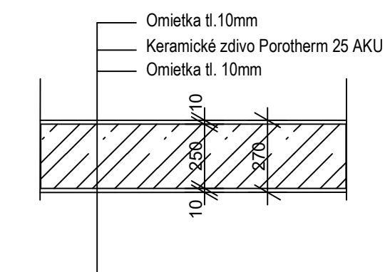
ST7- nosná zdená vnútorná stena
