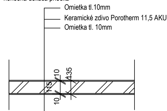
ST2- nenosná deliaca priečka
