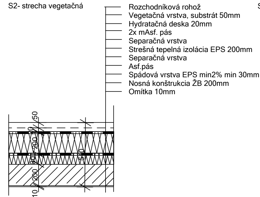
S2- strecha vegetačná
