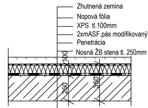
ST1- stena v 1.PP pod úrovňou terénu
