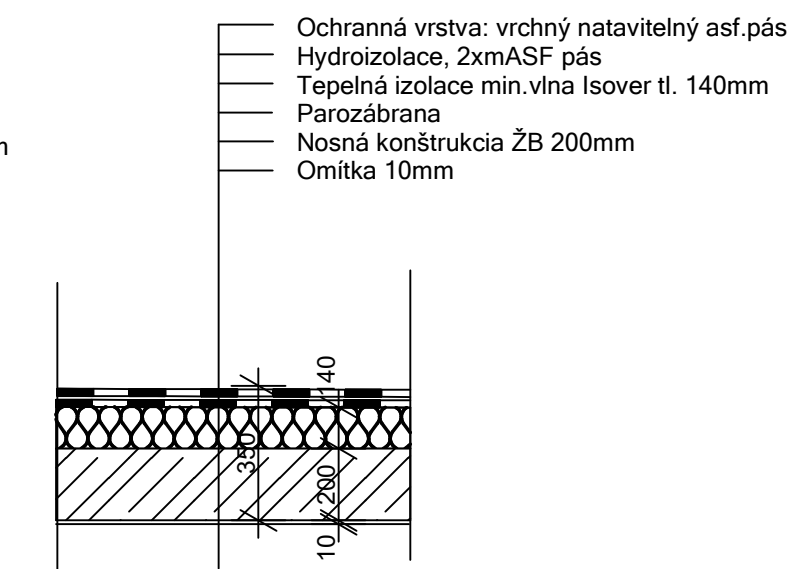
S3- strecha nepochozia
