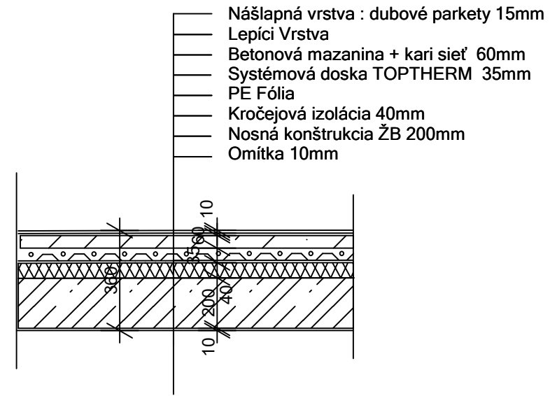
P2- Podlaha v obytných miestnostach s podlahovým vytápaním
