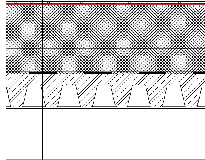
Skladba střechy
