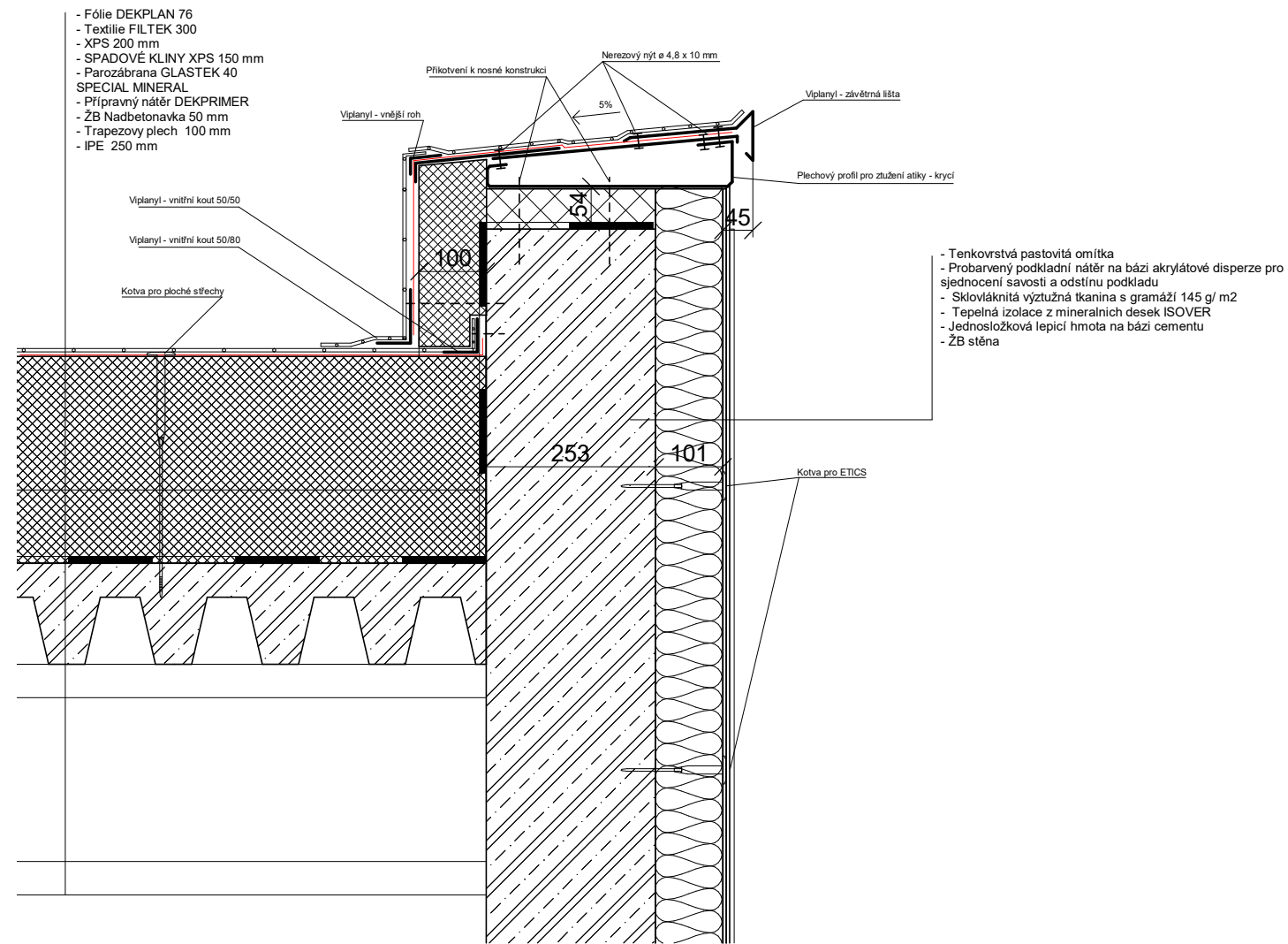
Detail atiky 1:10
