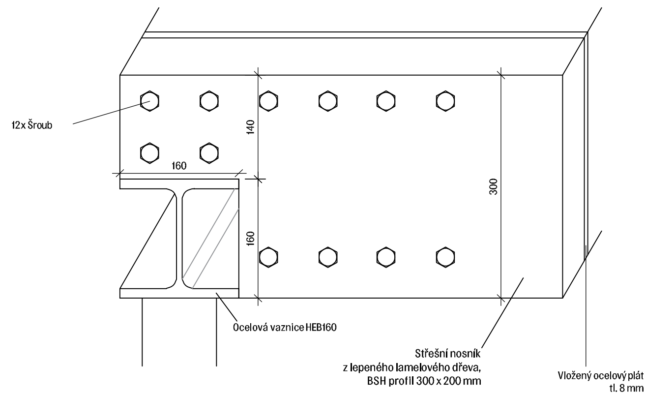
Napojení dřevěného vazníku a ocelové vaznice
