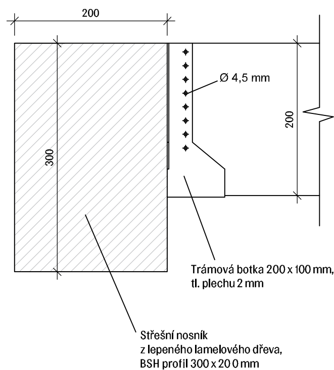
Napojení dřevěného vazníku a dřevěné krokvíčky
