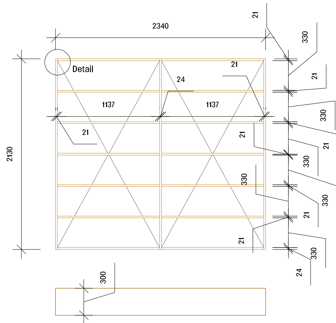
Pohled, půdorys 1:25
