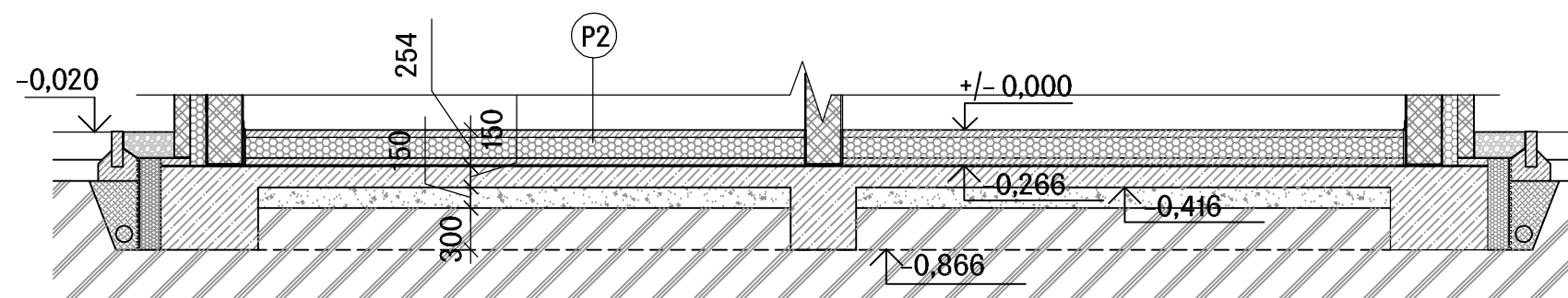
Řez A-A' 1:50
