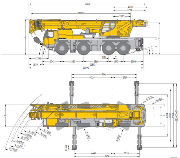
Mobilní jeřáb Liebherr LTM 1090-4.2
