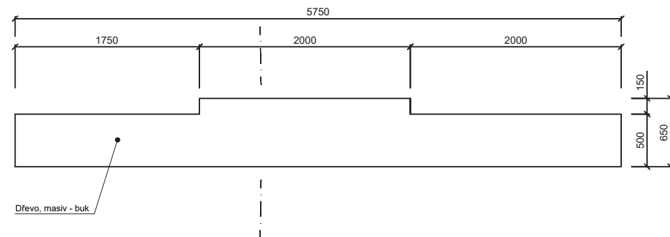
Řez M 1:50
