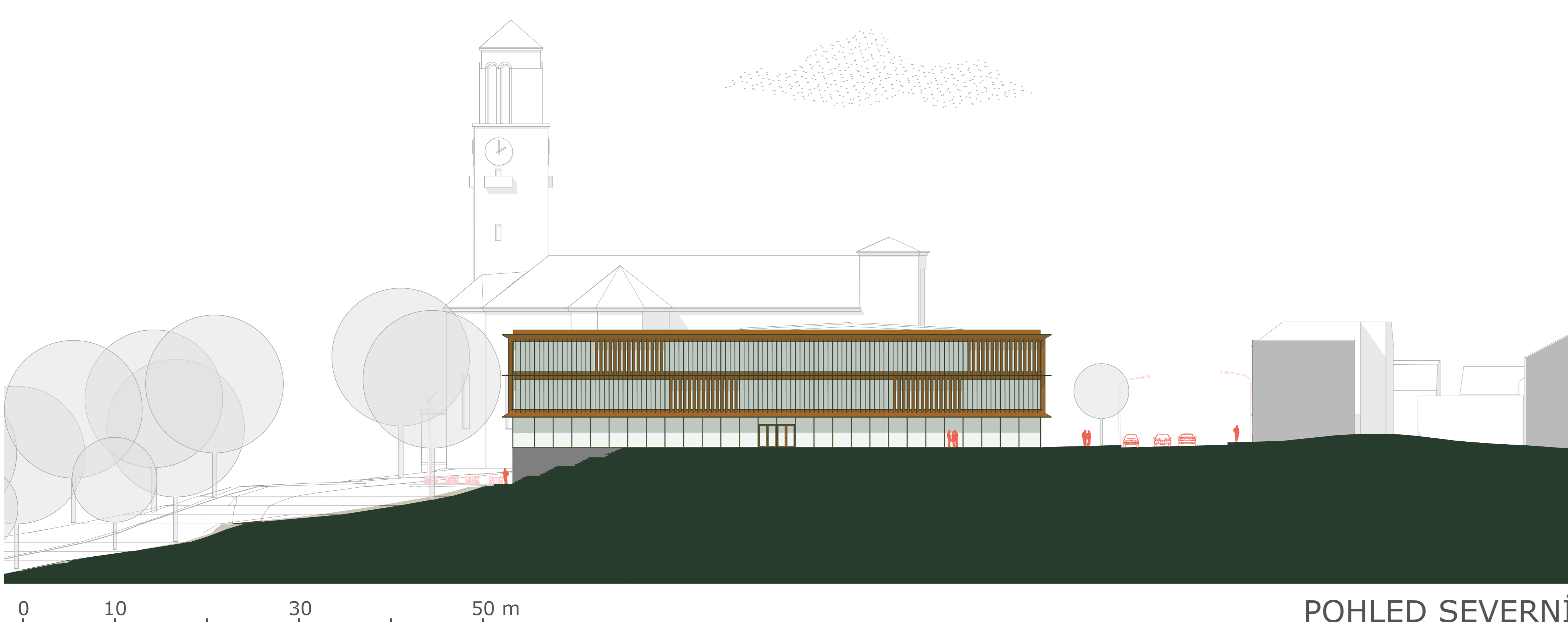
POHLED SEVERNÍ
