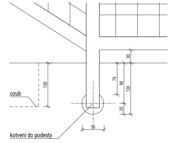
Detail ukotvení do podesty 1:5
