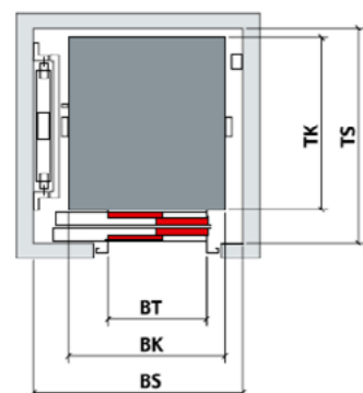
Kabina s jedním vstupem
