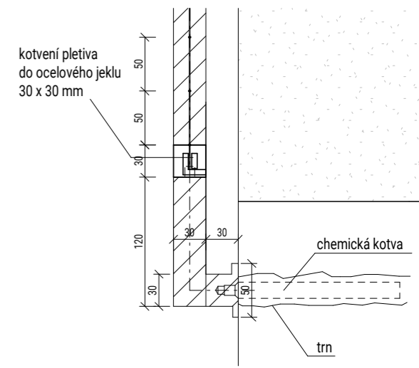
Řez ukotvením do podesty 1:5
