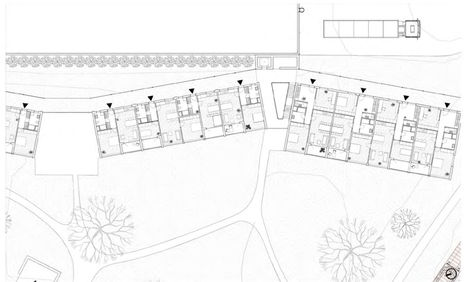
TYPICKÉ PODLAŽÍ M_1:200
