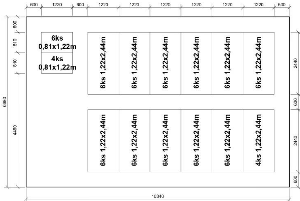
Obrázok 11 - Schéma skladovania vodorovného debnenia
