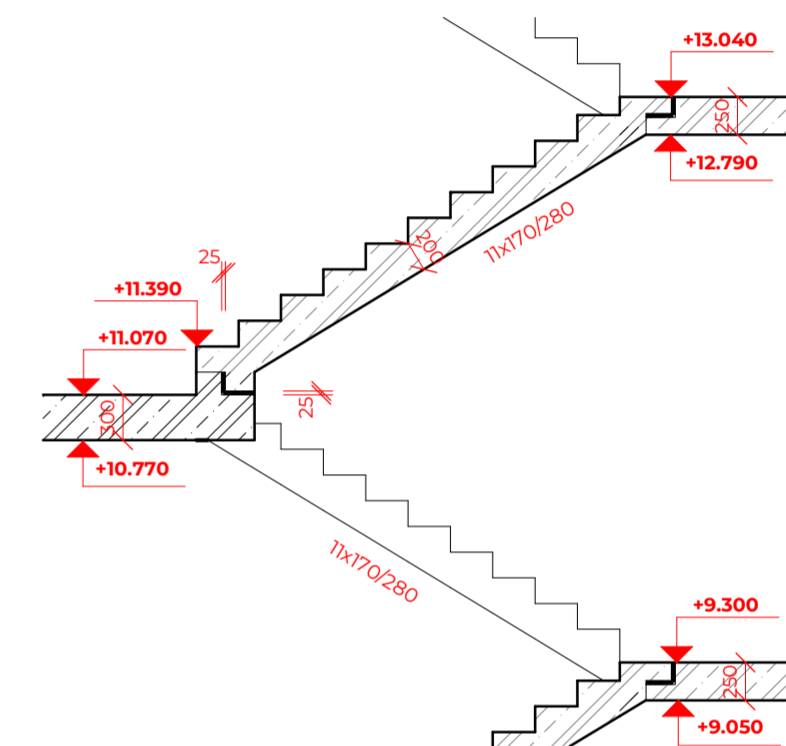
REZ SCHODISKOM M 1:50
