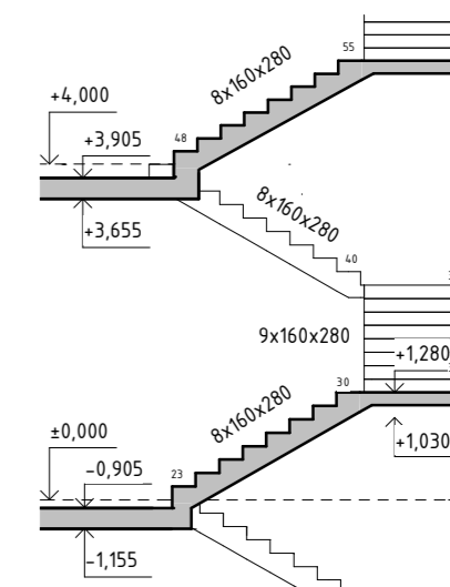
ŘEZ A-A'
