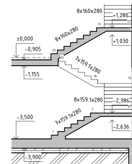
ŘEZ A-A'
