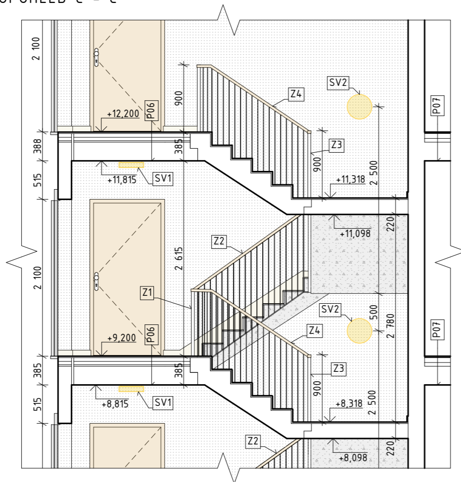
ŘEZOPHLED C - C'
