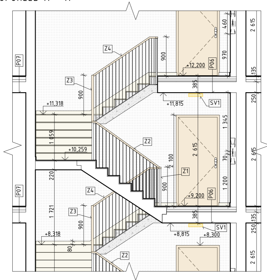
ŘEZOPHLED A - A'
