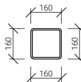
7) třmínek 25x8 délky 640 mm
