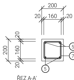
ŘEZ A-A'
