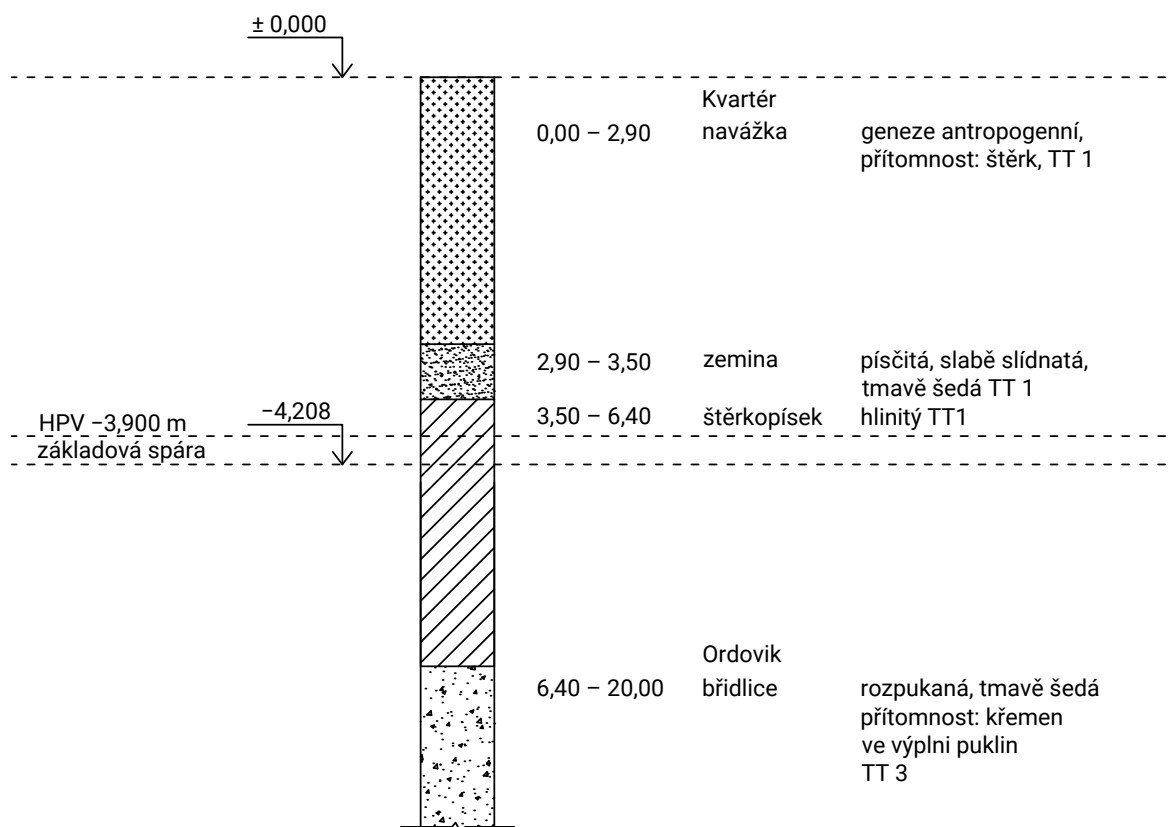
Obrázek B.2 – Půdní profil vrtu č. 580523
