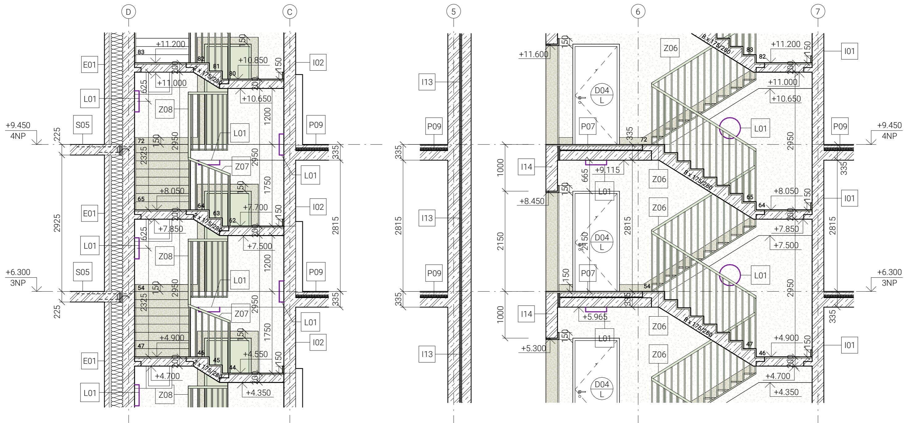
ŘEZOPHLED C-C'
