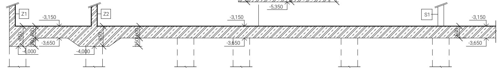
ŘEZ C-C'
