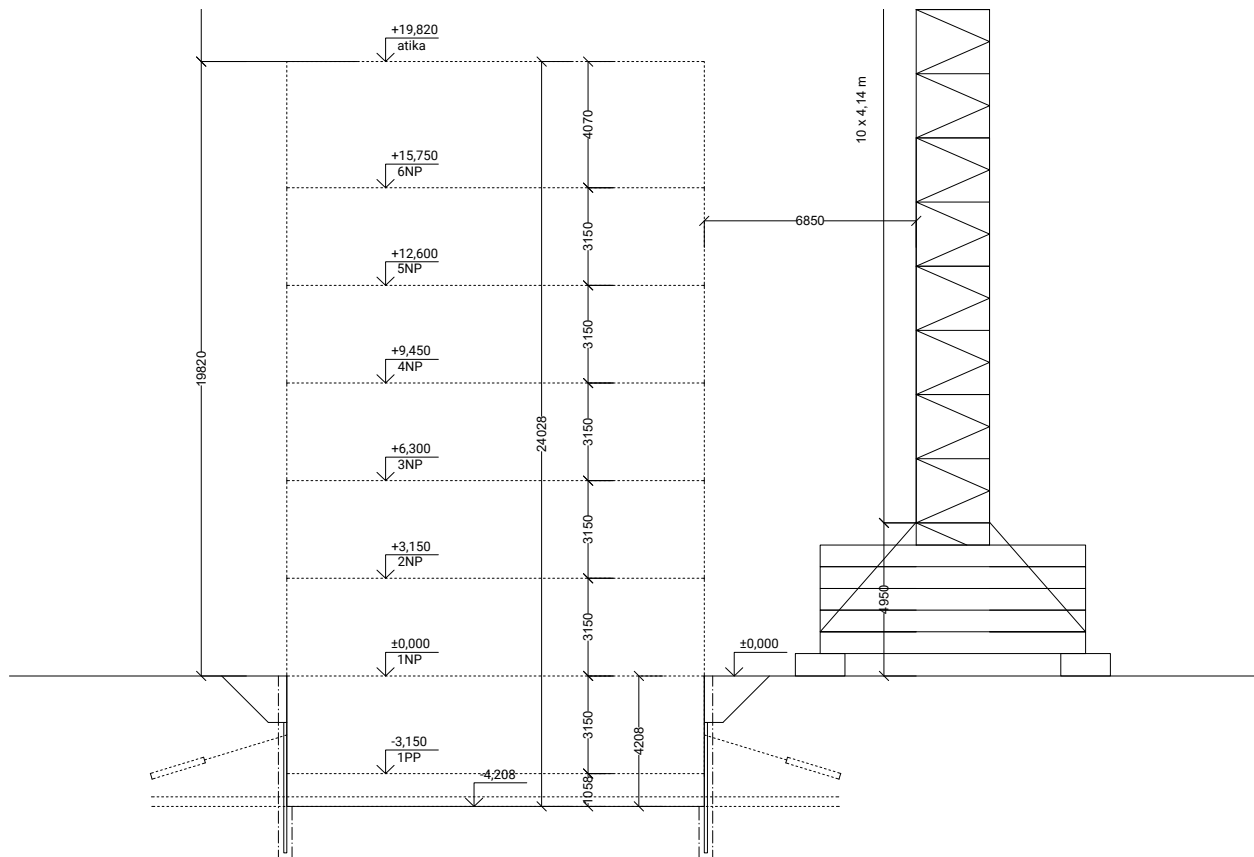
Schéma řezu stavební jámou
