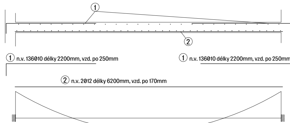
ŘEZ AA'
