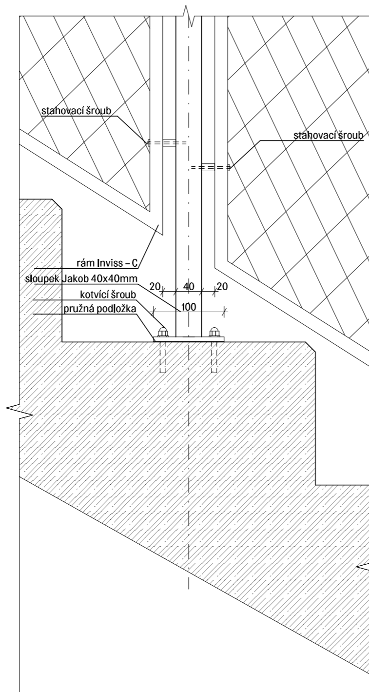
DETAIL KOTVENÍ M 1:4
