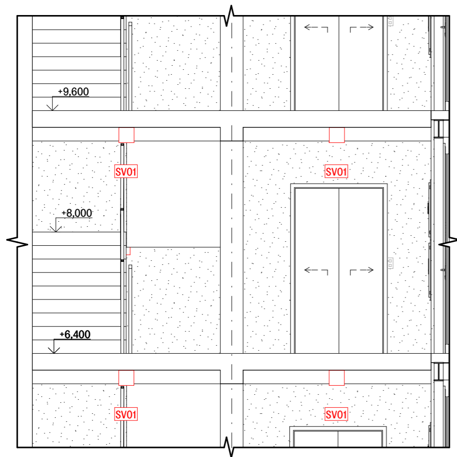
ŘEZOPHLED FF'
