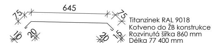
K4 - Oplechování atiky
