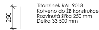
K5 - Krycí plech soklu
