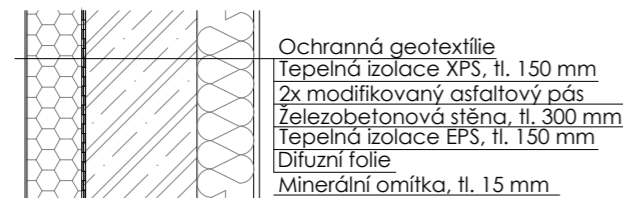
S6 - Exteriérová nosná stěna pod terénem
