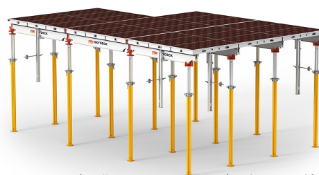
Obr. č. 1 - panelové stropní bednění PERI Skydeck
