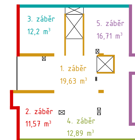
Obr. 4: Schemata betonářských záběrů
