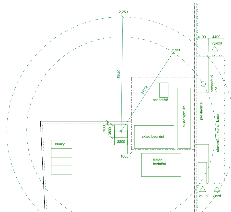
Obr. 13: Dosah výložníku jeřábu
