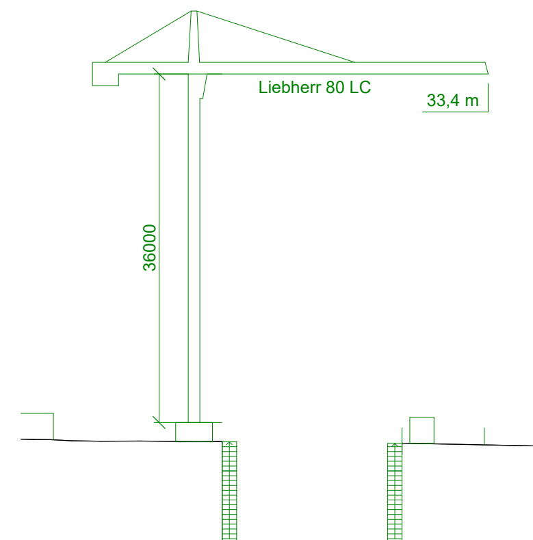
Obr. 12: Schema jeřábu, pohled
