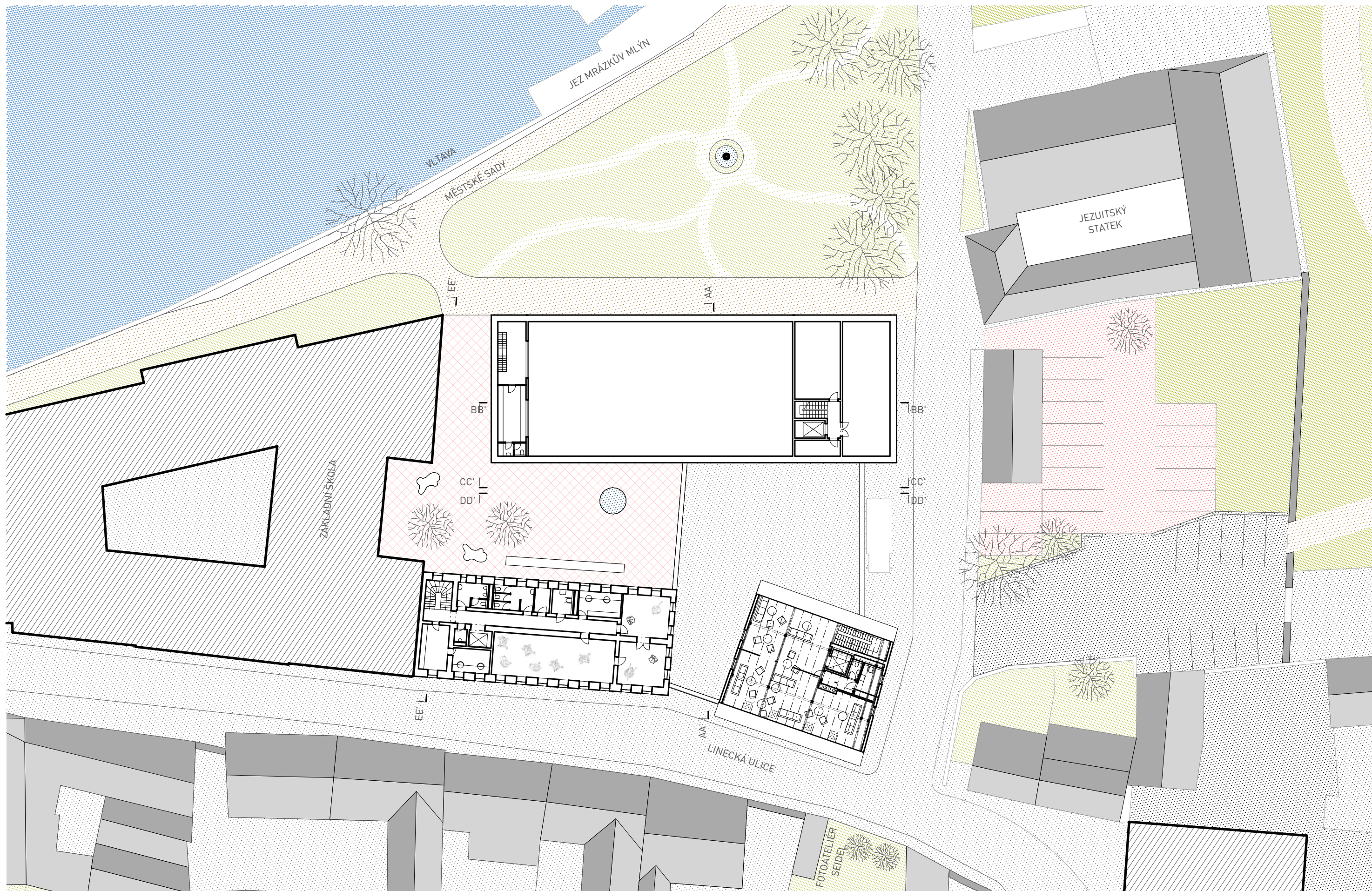
PŮDORYS 3.NP M 1:400
