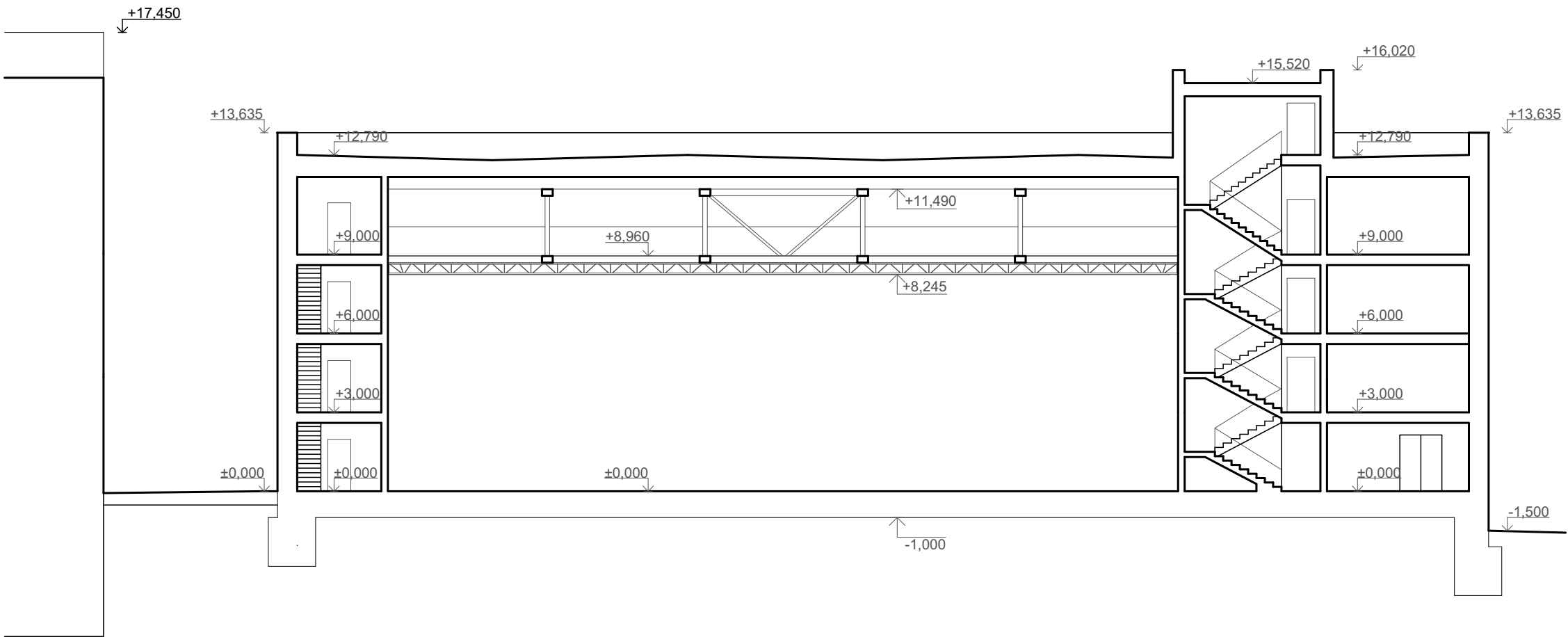
ŘEZ A-A' PODÉLNÝ M 1:200
