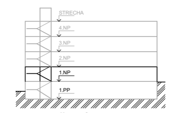
DETAIL ULOŽENÍ PREF. RAMENE
