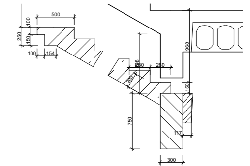
DETAIL ULOŽENÍ PREF. RAMENE
