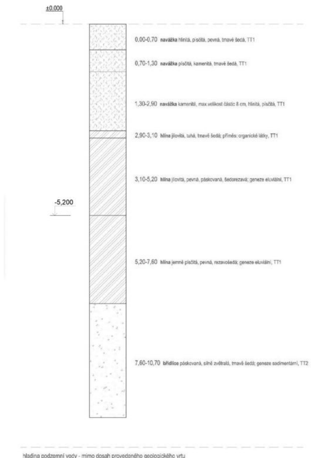
Schéma geologického vrtu
