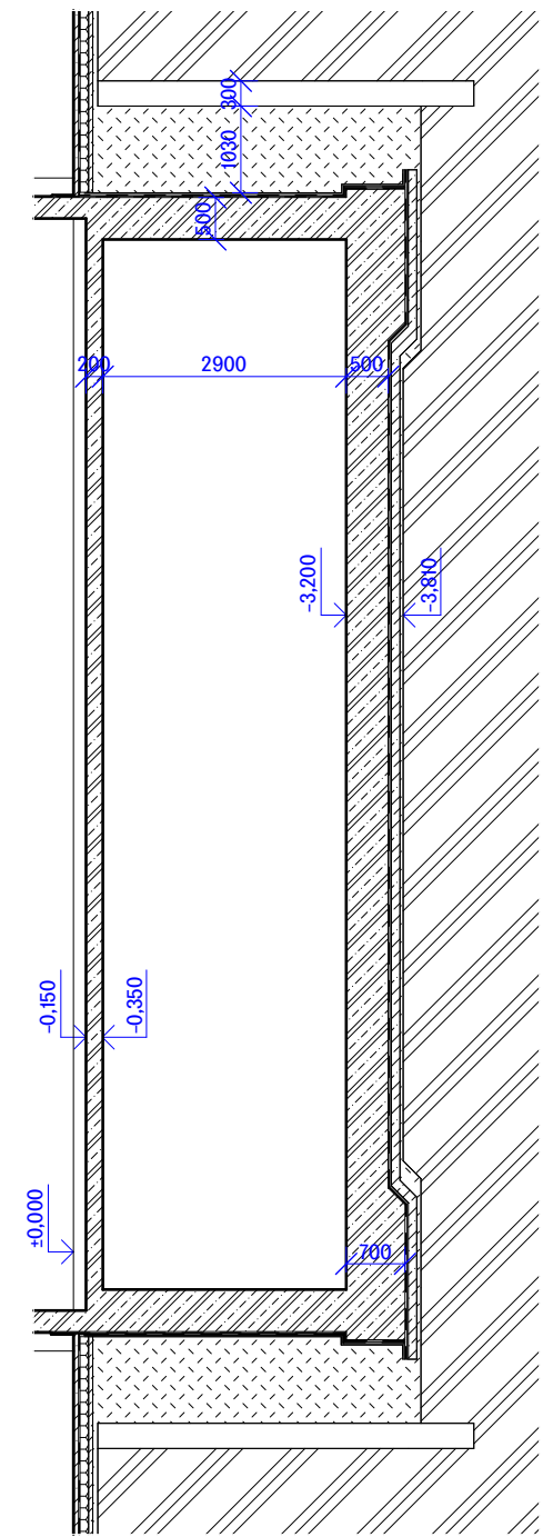
ŘEZ B-B'
