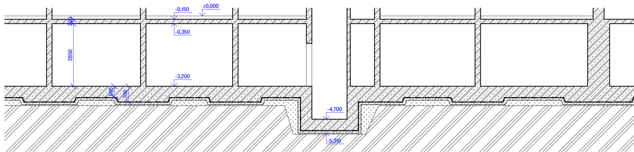
ŘEZ A-A'
