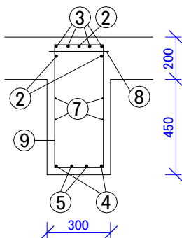
ŘEZ B-B' 1:25
