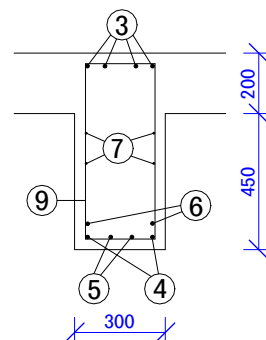
ŘEZ A-A' 1:25
