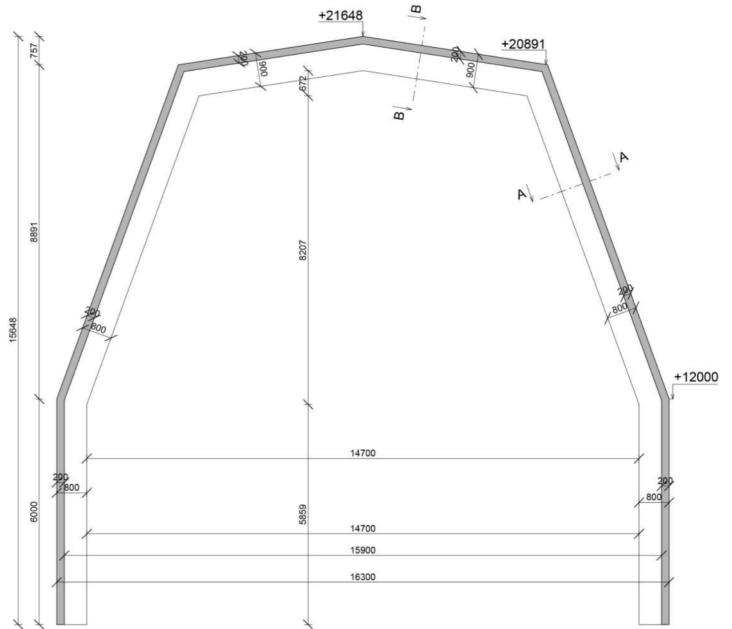
Řez A-A
