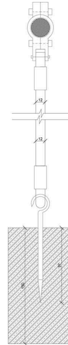
Detail kotvení lána M 1:50
