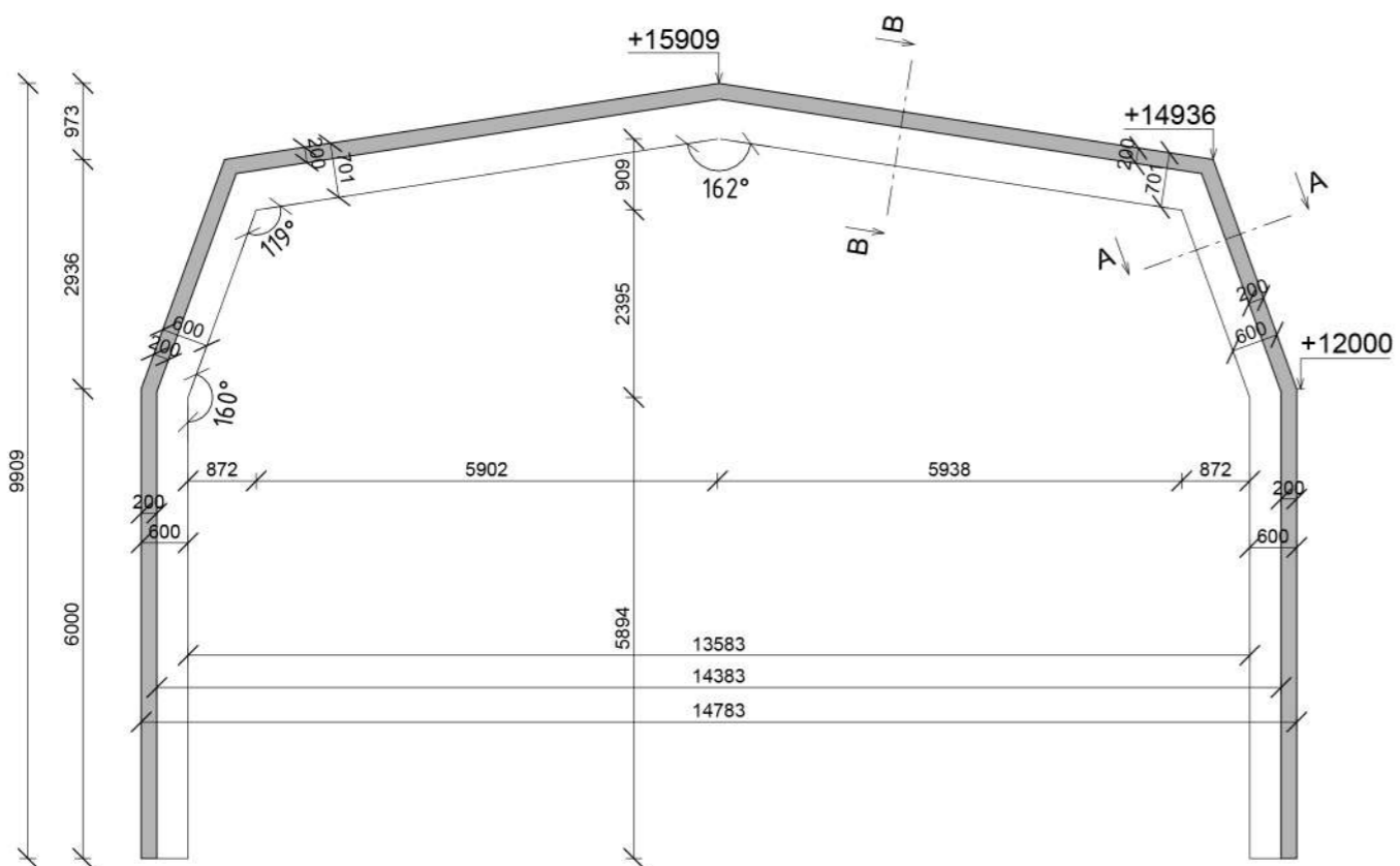
Řez A-A
