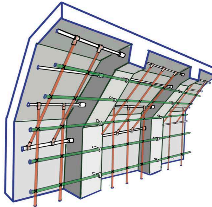
Perspektivní skica systému lán
