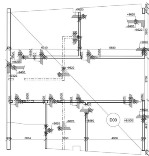
Výkres tvaru nad 1.NP
