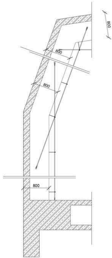
Detail kotvení svislých lán M 1:50
