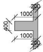
Řez B-B
