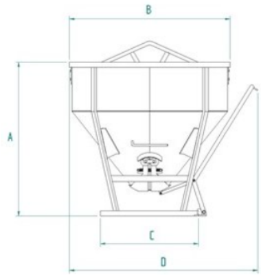
Obr. Betonářský koš Boscaro C-99
