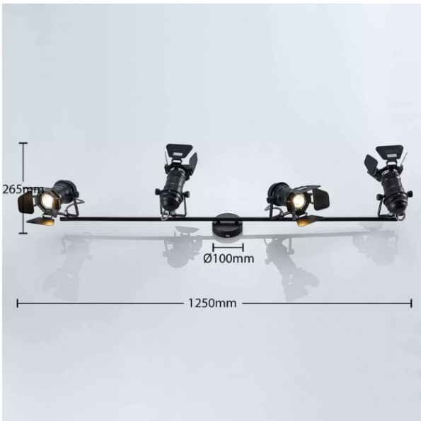
Stropní bodové osvětlení Tilen, 4zdrojové
