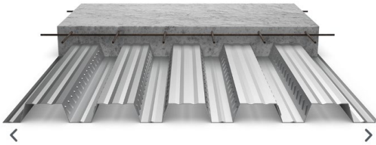
Obr. Bednění Cofrasol 55/250
