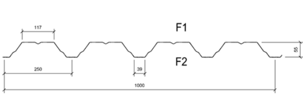
Obr. Schématický řez trapézovým plechem
