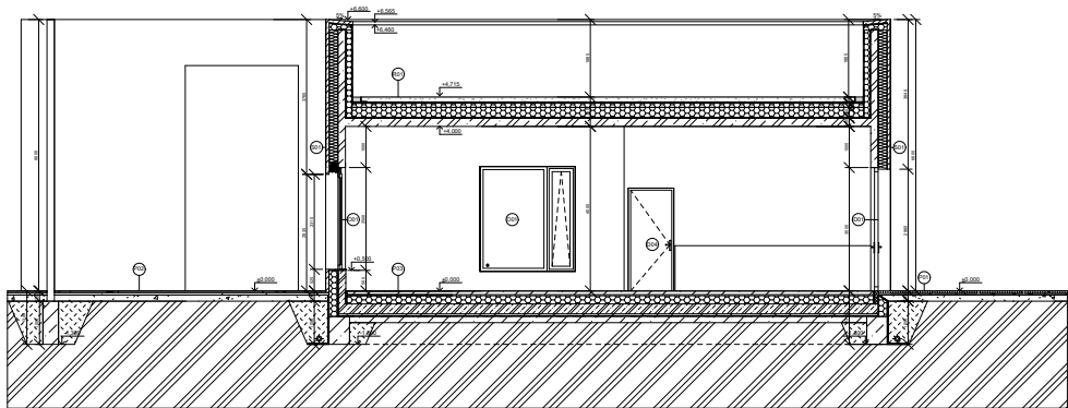
ŘEZ C - C'
