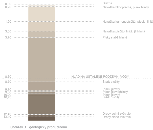
Obrázek 3 - geologický profil terénu
