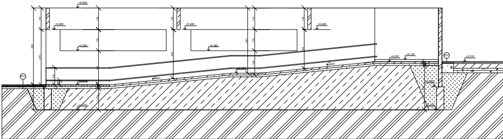
ŘEZ B - B'
