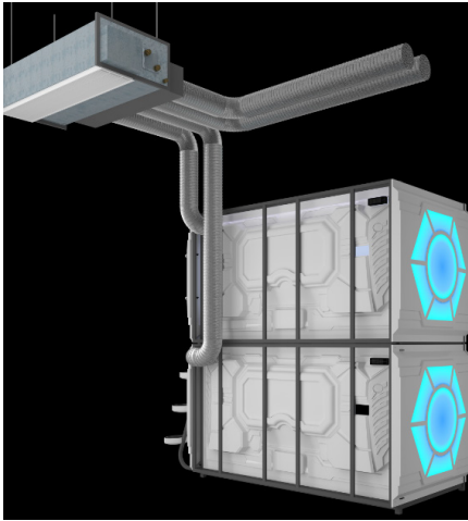
detaili napojení kapslové postele na VZT jednotku zdroj: korespondence s prodejcem přes Alibaba.com
