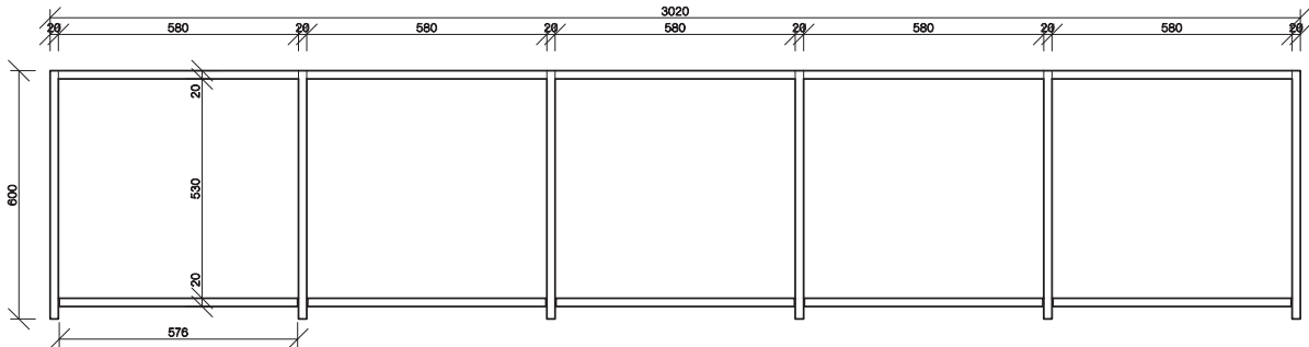
půdorysný řez ve výšce 300mm (1 : 20)
