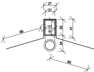
řez příčný (1 : 5)
