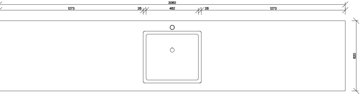
půdorys (1 : 20)
