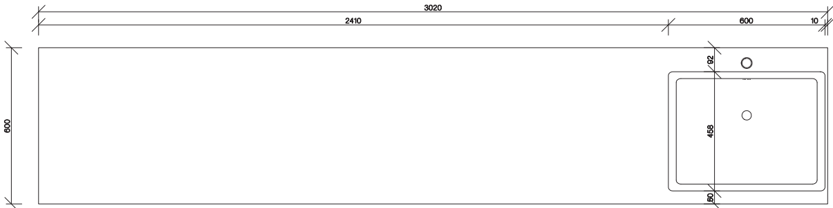
půdorys (1 : 20)
