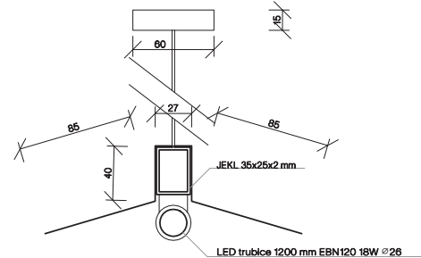
řez příčný (1 : 5)
