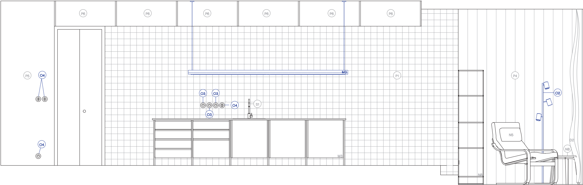
pohled A-A'
