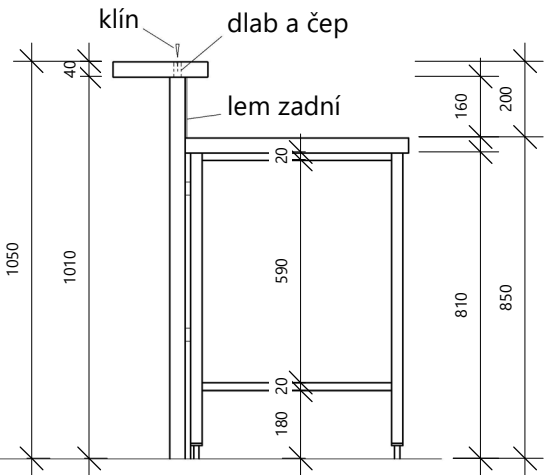
ŘEZ A-A'
