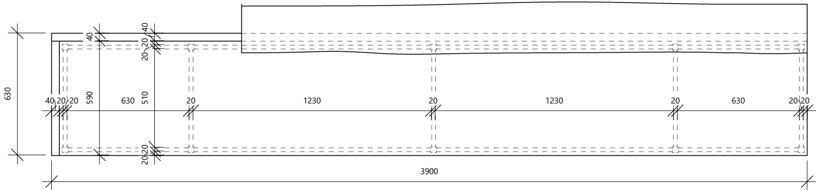
PŮDORYS
