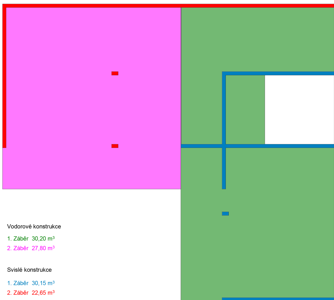
Obrázek D.5.2: Betonářské záběry
