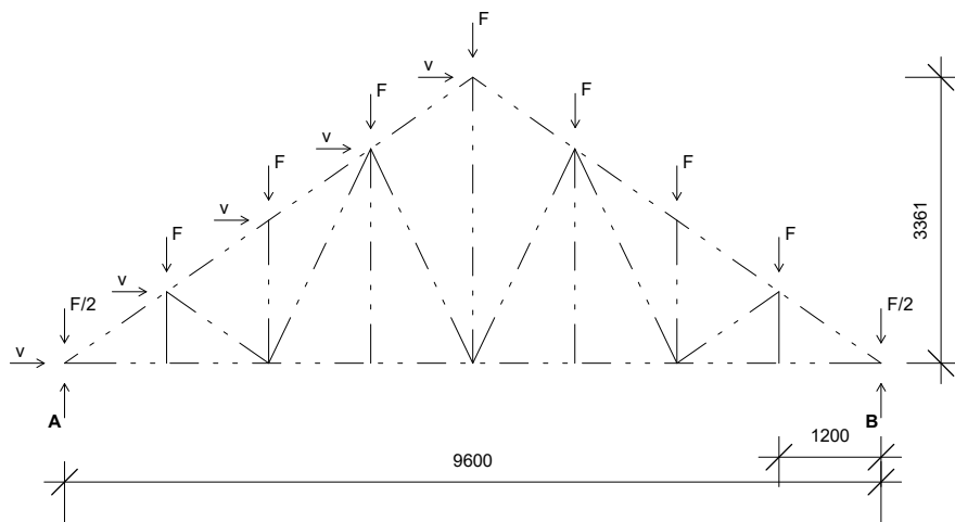
Obrázek D.2.2: Schéma vazníku
