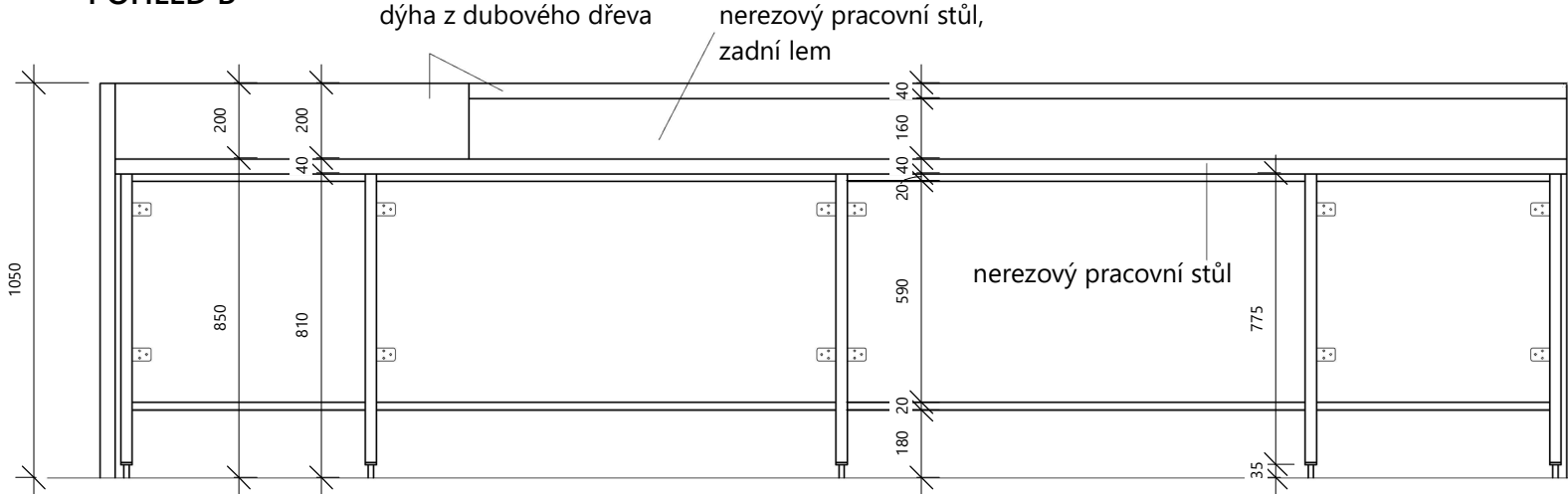
POHLED B
