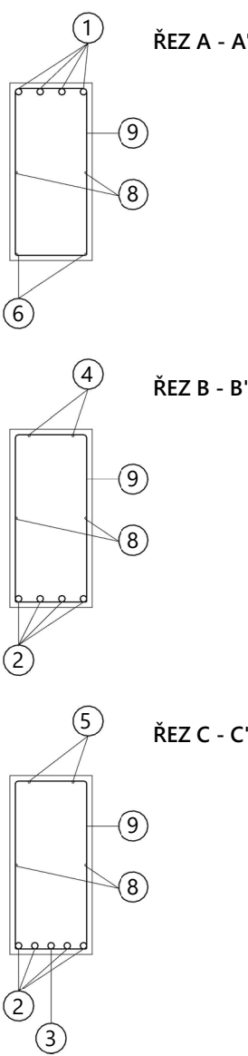
ŘEZ PŘÍČNÝ 1:25
