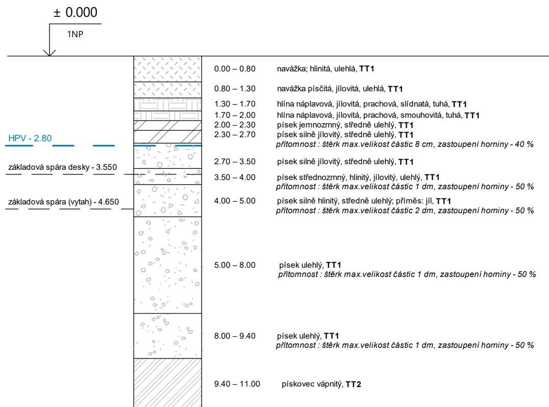
Obrázek D.2.1: Půdní profil
