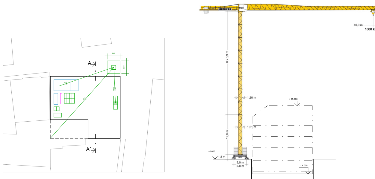
Obrázek D.5.8: Výkres půdorysu a řezu jeřábem na pozici ve staveništi
