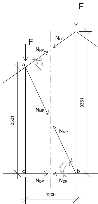
Obrázek D.2.3: Síly působící na vazníku
