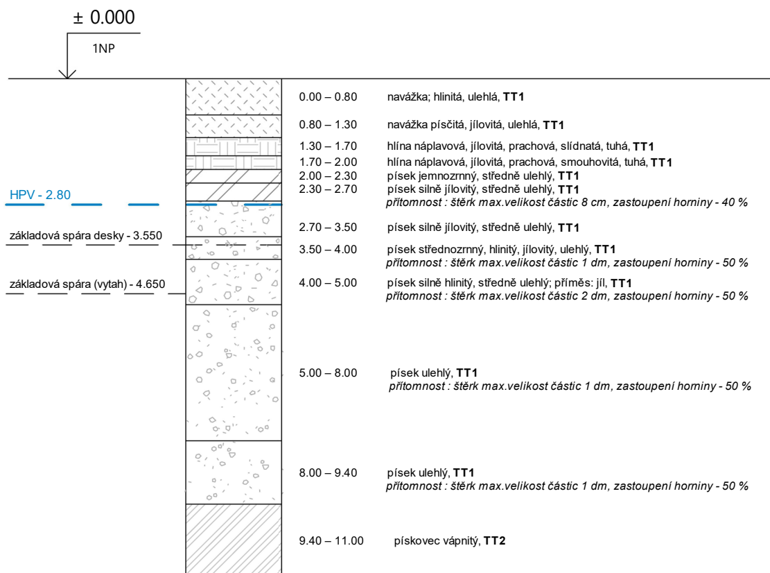
Obrázek D.5.1: Půdní profil
