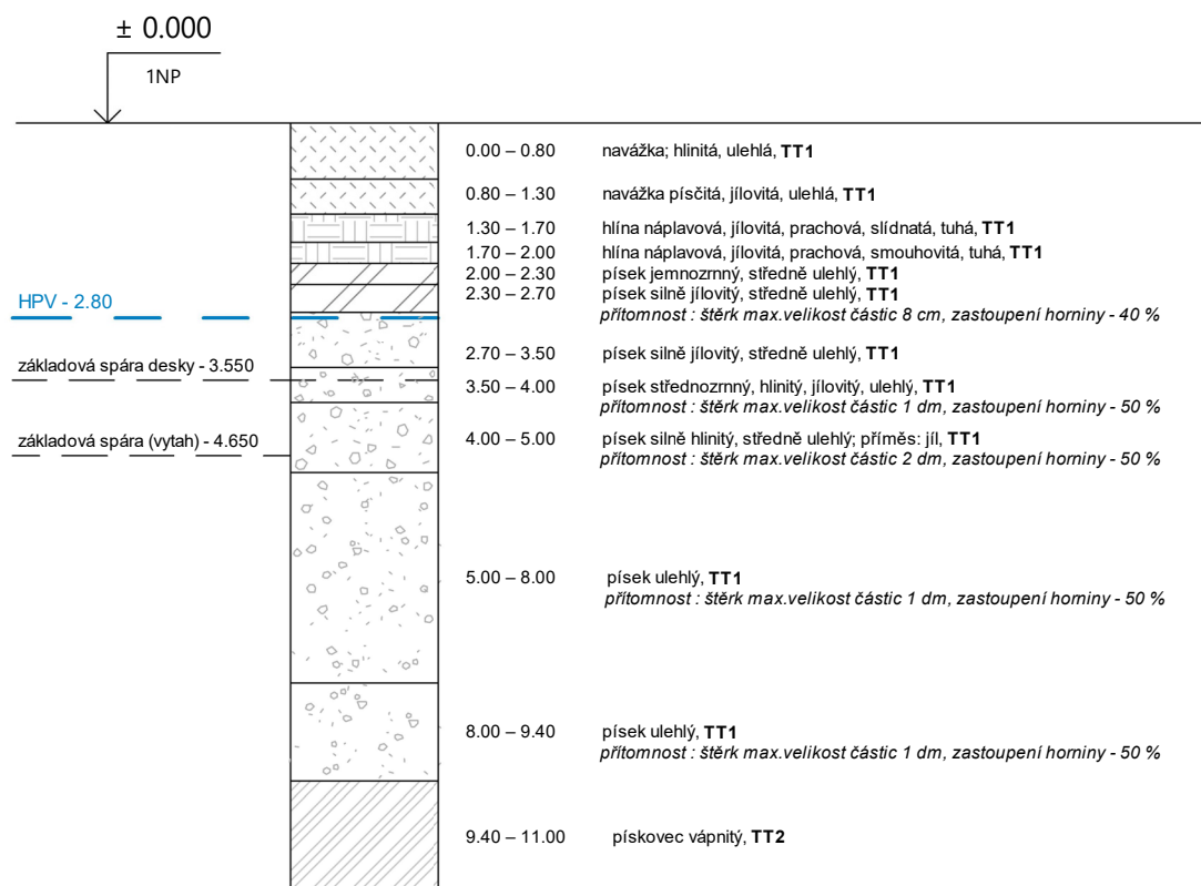
Obrázek B.1.1: Půdní profil
