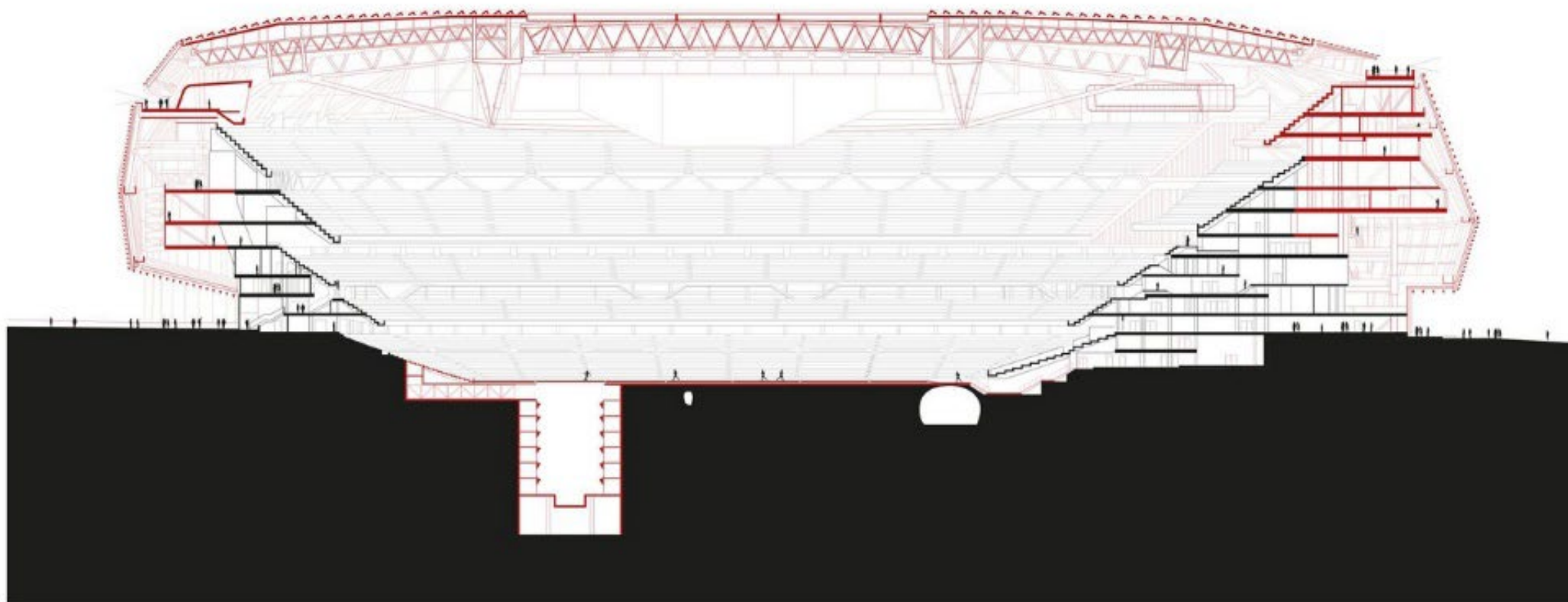
Querschnitt | Maßstab 1:1000
